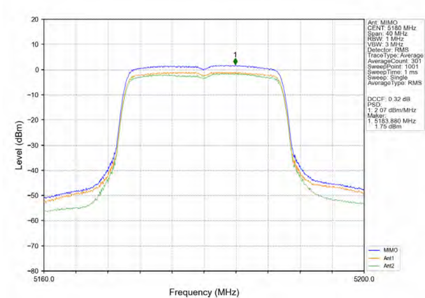
802.11ax(HEW20) LCH 5180MHz RU242 Left MIMO NTN
