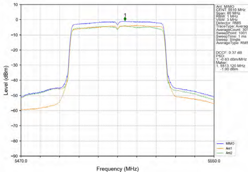
802.11ax(HEW40) LCH 5510MHz RU484 Left MIMO NTNW
