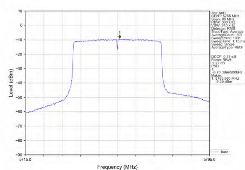
802.11ax(HEW40) LCH 5755MHz RU484 Left Ant1 NTN
