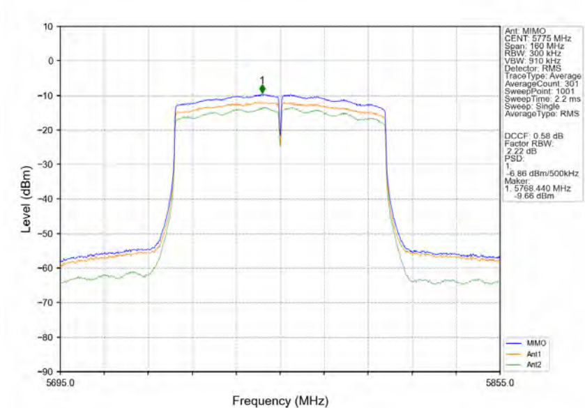
802.11ac(VHT80) MCH 5775MHz MIMO NTN
