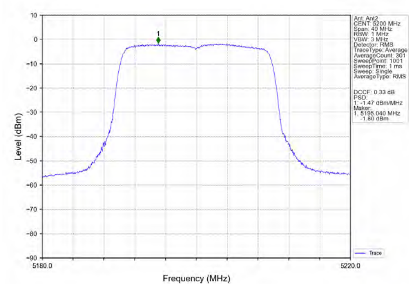
802.11ax(HEW20) MCH 5200MHz RU242 Left MIMO NTNW
