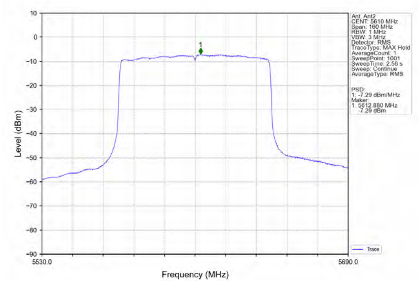
802.11ax(HEW80) HCH 5610MHz RU996 Left MIMO NTN
