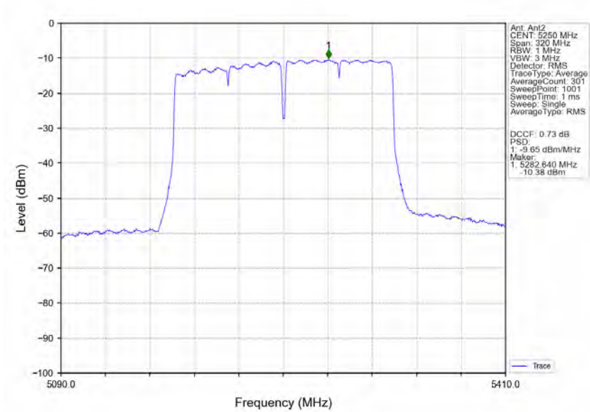
802.11ac(VHT160) MCH 5250MHz MIMO NTN
