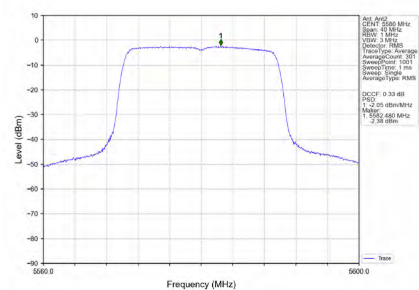
802.11ax(HEW20) MCH 5580MHz RU242 Left MIMO NTNW
