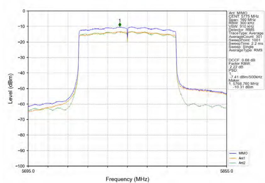
802.11ax(HEW80) MCH 5775MHz RU996 Left MIMO NTNW
