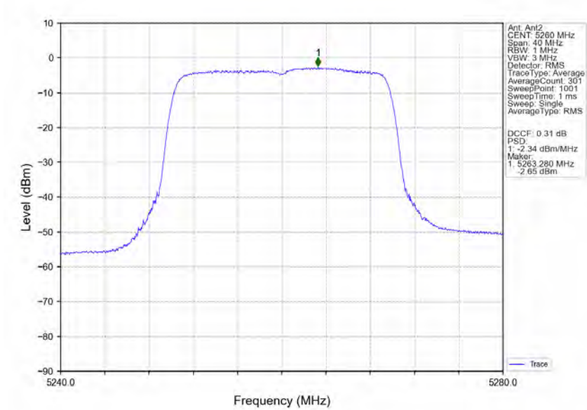
802.11ax(HEW20) LCH 5260MHz RU242 Left MIMO NTN
