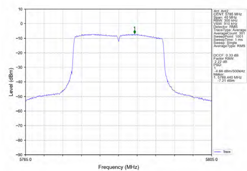
802.11ax(HEW20) MCH 5785MHz RU242 Left MIMO NTNW
