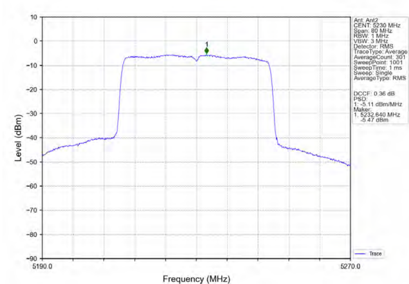
802.11ax(HEW40) HCH 5230MHz RU484 Left Ant2 NTN
