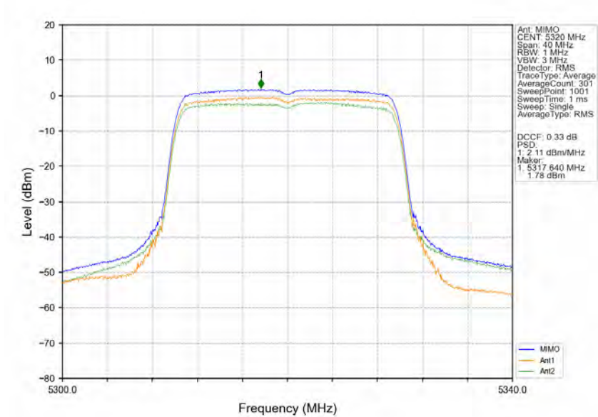
802.11ax(HEW20) HCH 5320MHz RU242 Left MIMO NTN
