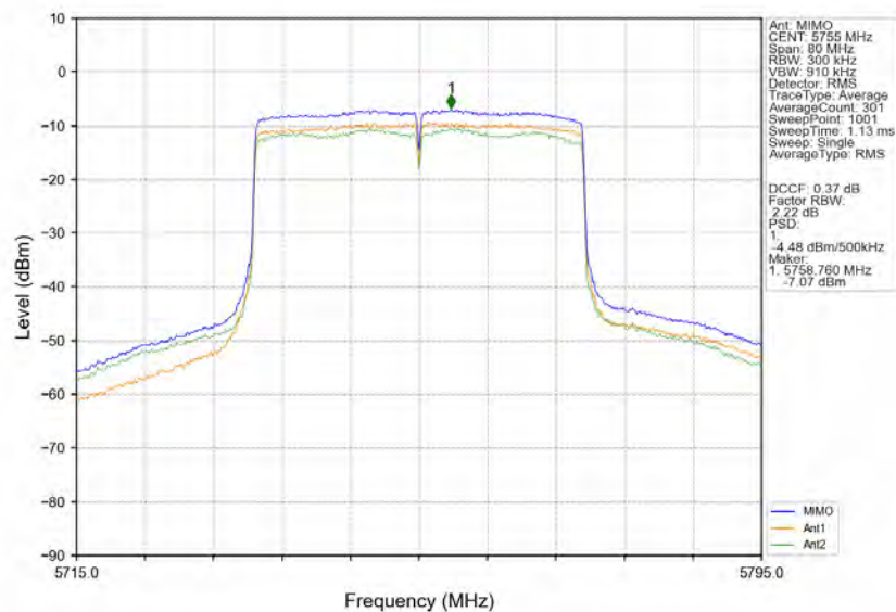
802.11ax(HEW40) LCH 5755MHz RU484 Left MIMO NTN
