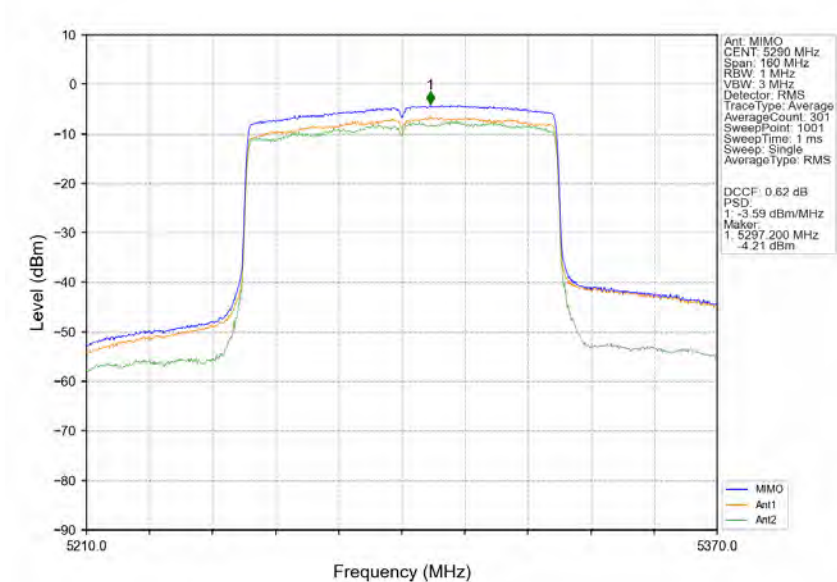
802.11ax(HEW80) MCH 5290MHz RU996 Left MIMO NTNW
