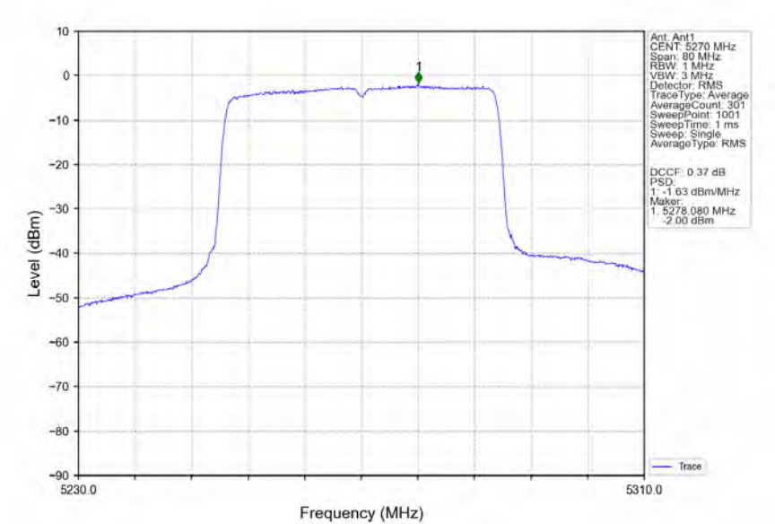
802.11ax(HEW40) LCH 5270MHz RU484 Left Ant1 NTN
