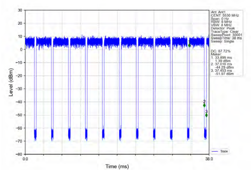
802.11ac(VHT80) LCH_5530MHz_Ant1_NTNV
