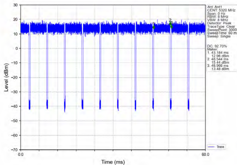
802.11ax(HEW20) HCH 5320MHz RU242 Left Ant1 NTNW
