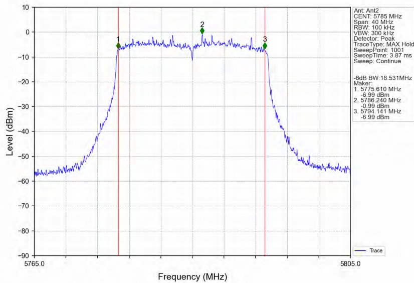
802.11ax(HEW20) MCH_5785MHz RU242 Left Ant2 NTNv
