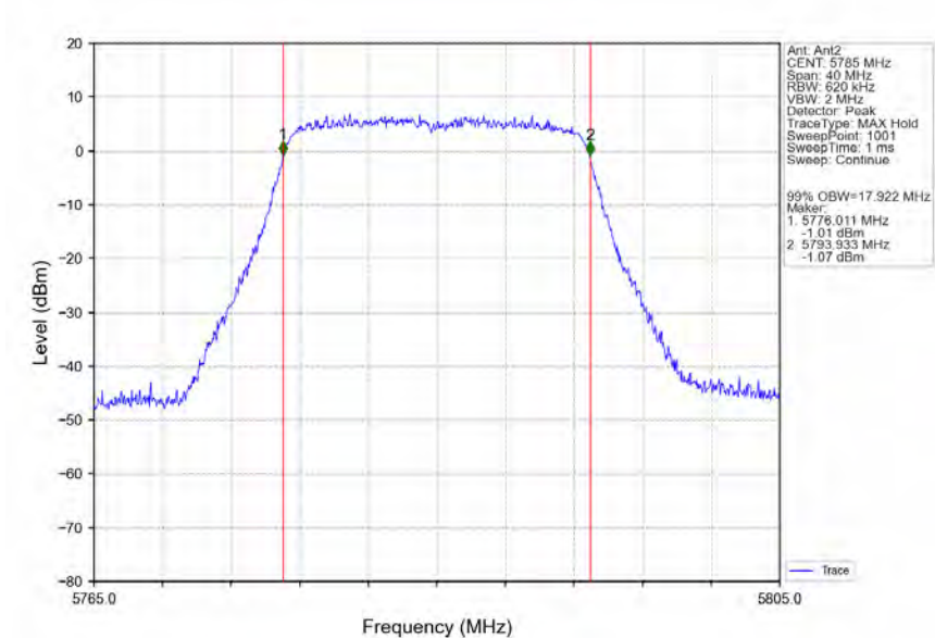
802.11ac(VHT20) MCH_5785MHz_Ant2_NTNV
