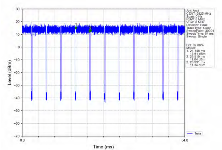
802.11ac(VHT20) HCH_5825MHz_Ant1_NTNV
