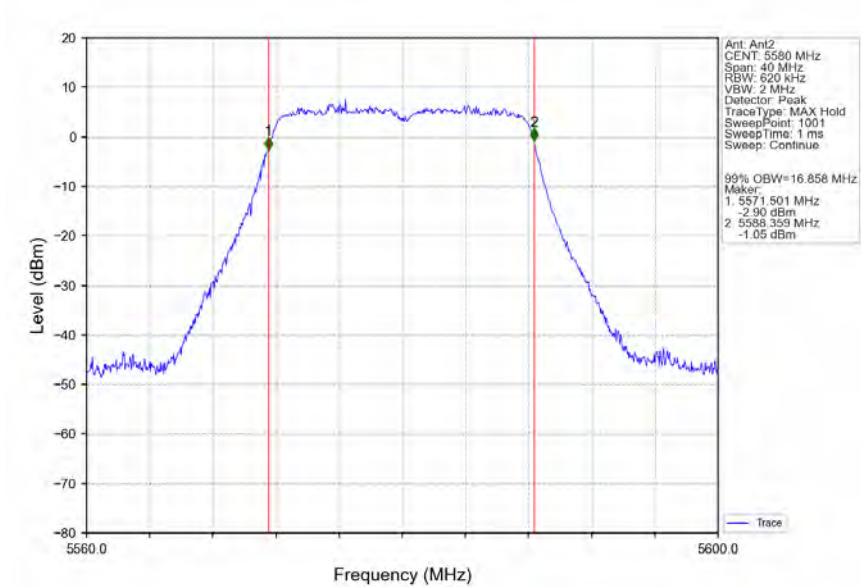
802.11a MCH_5580MHz_Ant2_NTNV
