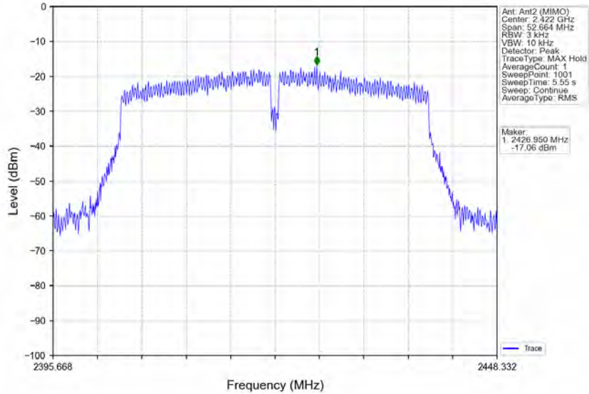
802.11n(HT40)_LCH_2422MHz_MIMO_NTNV
