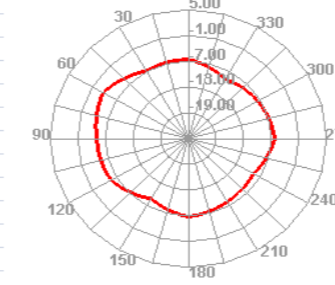
2500.000MHz E2
