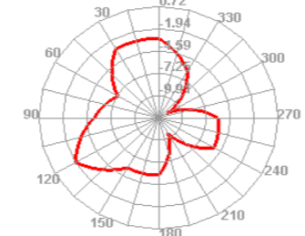
2450.000MHz E2
