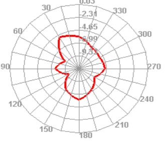
2400.000MHz E1
