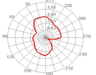
2450.000MHz E1
