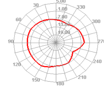
2400.000MHz E2
