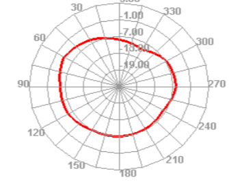
2450.000MHz H
