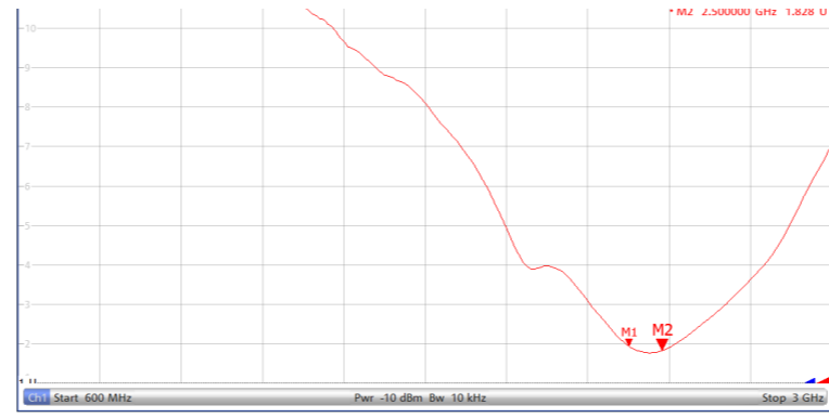
2450.000MHz H
