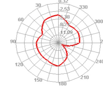
2500.000MHz E1
