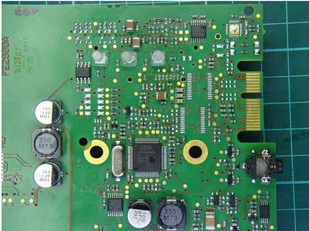
(101) EUT Photo (M/N: BIS U-626-069-111-06-ST32)
