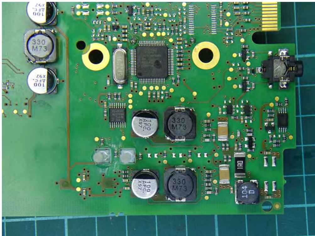
(102) EUT Photo (M/N: BIS U-626-069-111-06-ST32)
