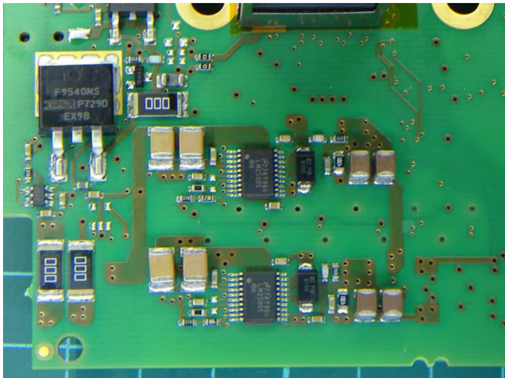
(72) EUT Photo (M/N: BIS U-626-069-111-06-ST31)
