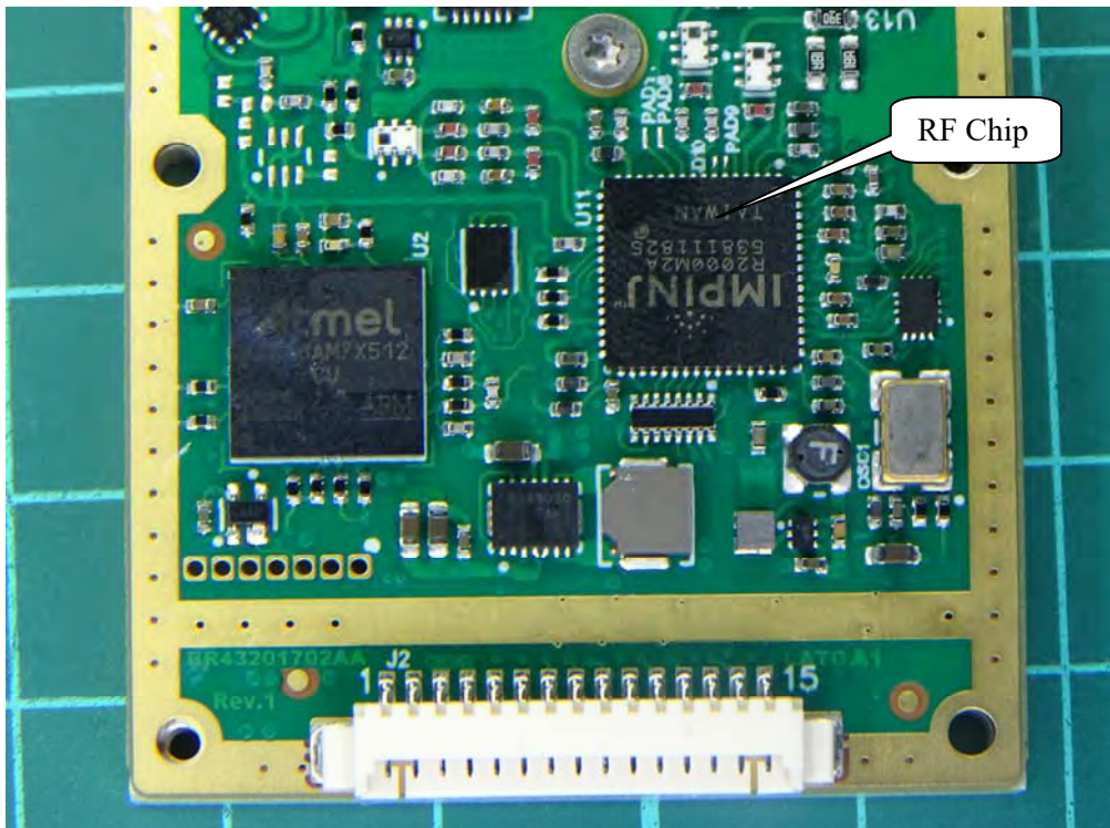
(94) EUT Photo (M/N: BIS U-626-069-111-06-ST32)
