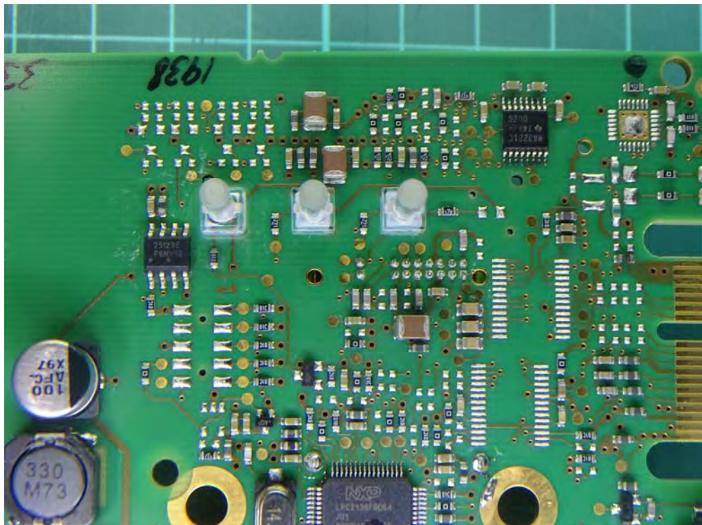
(74) EUT Photo (M/N: BIS U-626-069-111-06-ST31)
