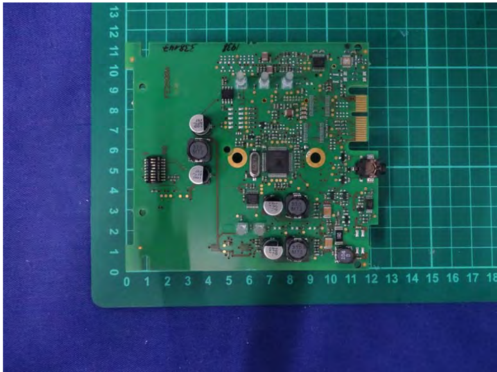
(73) EUT Photo (M/N: BIS U-626-069-111-06-ST31)
