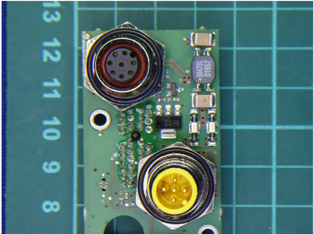
(83) EUT Photo (M/N: BIS U-626-069-111-06-ST32)
