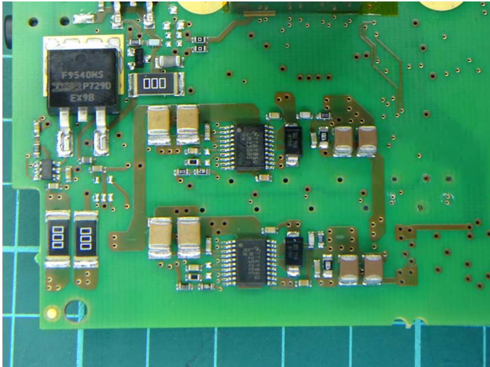
(99) EUT Photo (M/N: BIS U-626-069-111-06-ST32)
