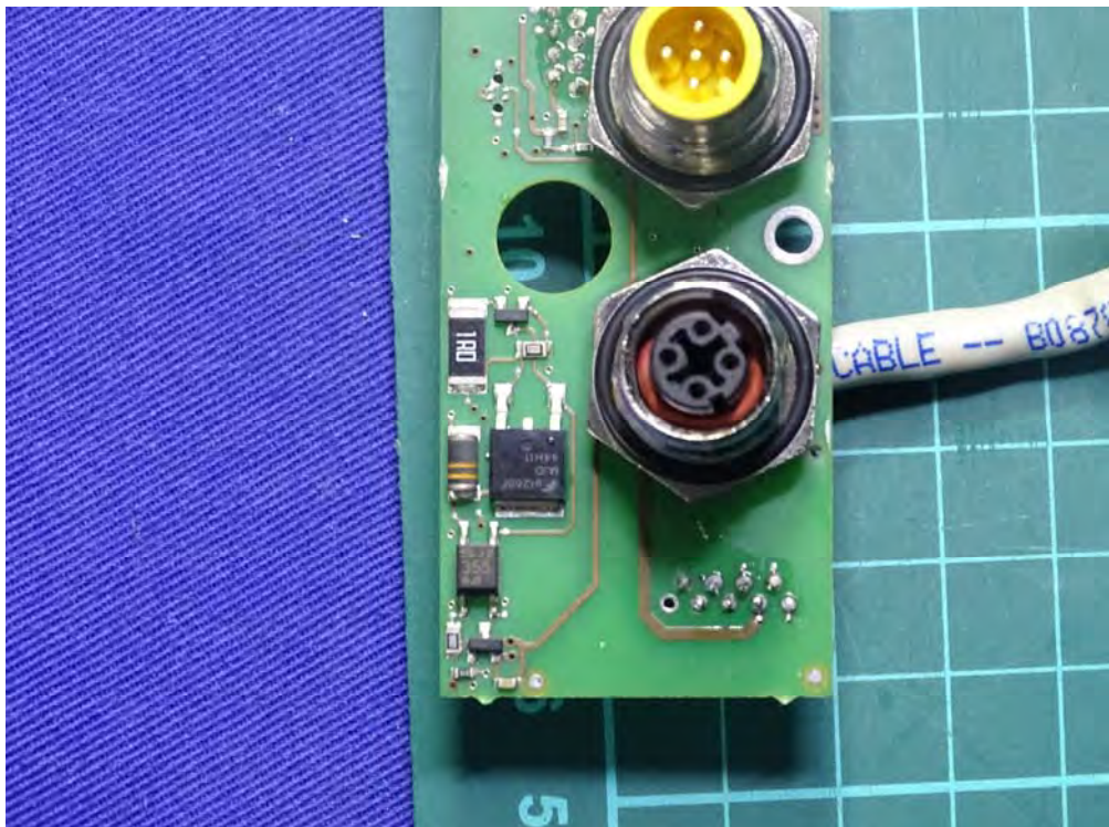
(84) EUT Photo (M/N: BIS U-626-069-111-06-ST32)
