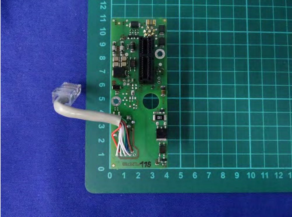
(79) EUT Photo (M/N: BIS U-626-069-111-06-ST32)
