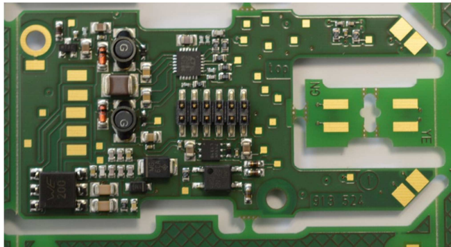
PCBA Bottom
