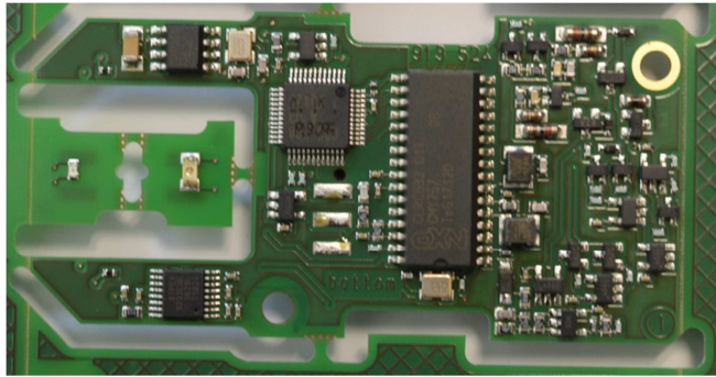
PCBA Top
