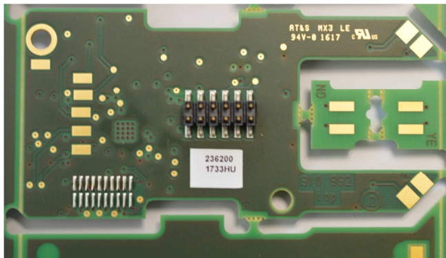
PCBA Bottom
