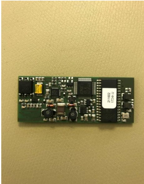
PCBA Top
