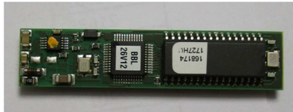
PCBA Top
