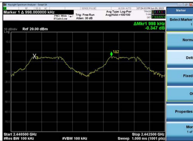
GFSK
