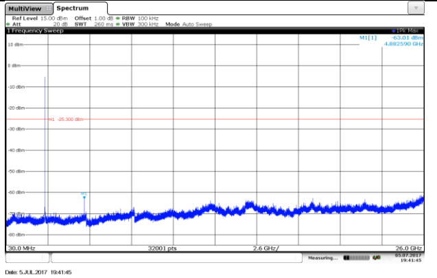
CH39 SE
