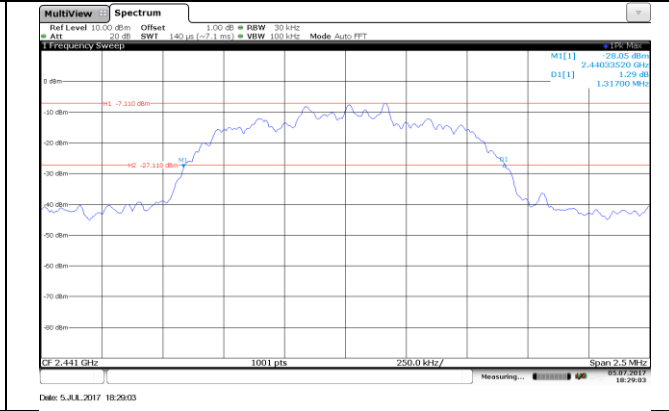
CH39
