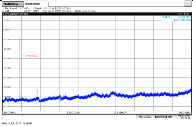
CH00 SE
