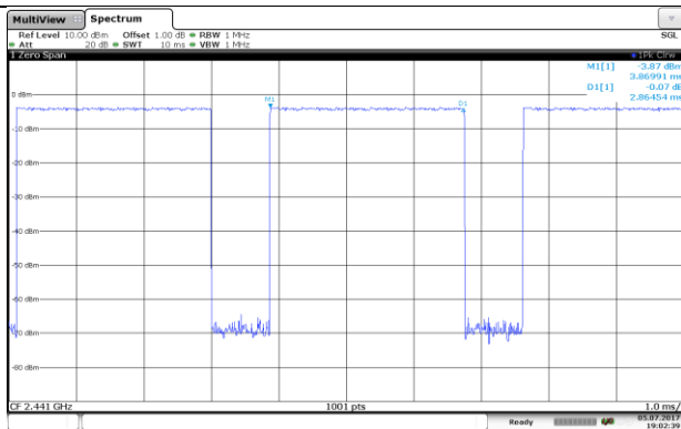
3-DH5
