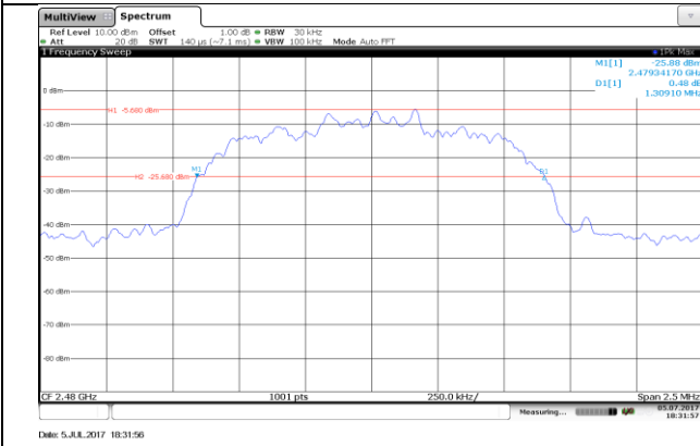
CH78
