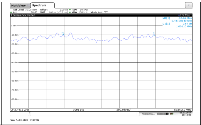
\pi/4 DQPSK
