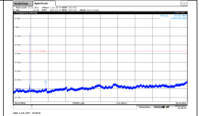
CH39 SE
