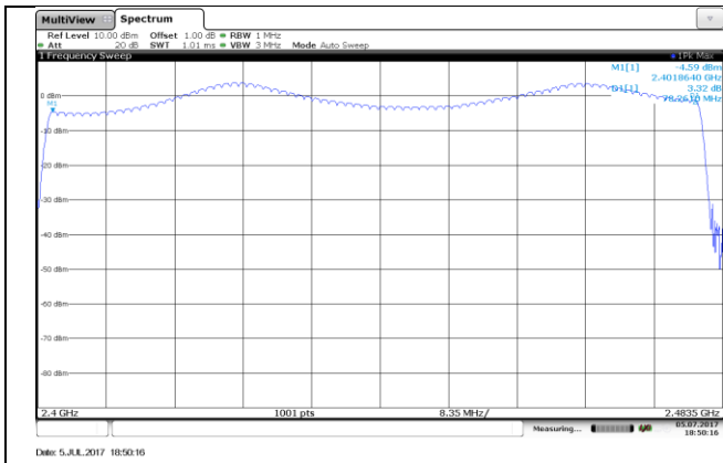
GFSK
