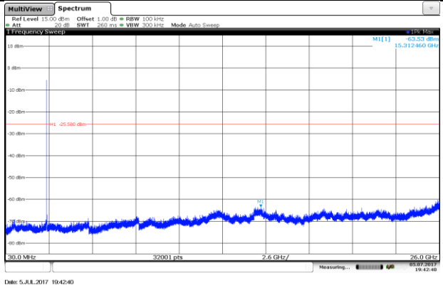
CH78 SE
