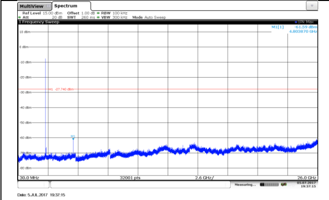
CH00 SE
