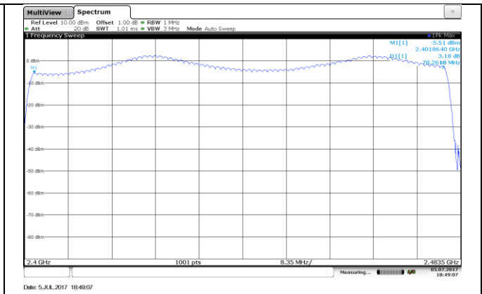
\pi/4 DQPSK
