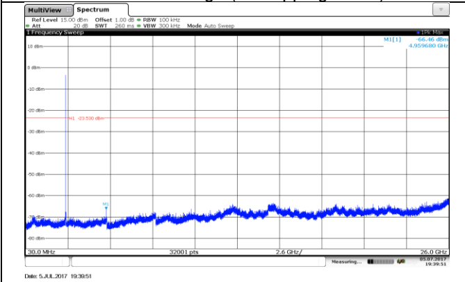
CH78 SE
