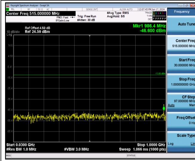
Band2-20MHz-QPSK-18700-1RB#0-Range1:30~1000MHz
