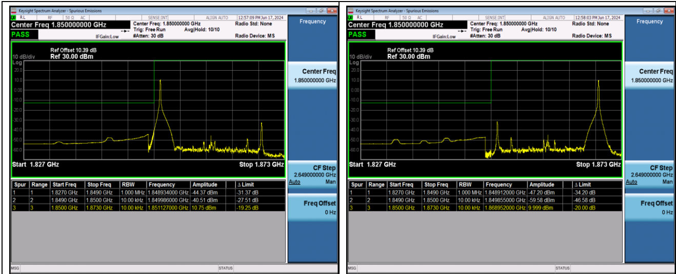
Band2-20MHz-QPSK-18700-100RB#0
