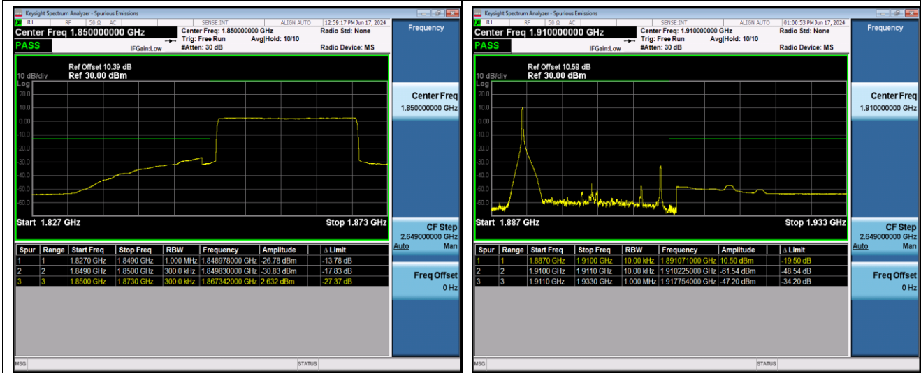
Band2-20MHz-QPSK-19100-1RB#99
