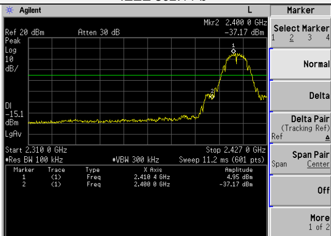
IEEE 802.11 b
