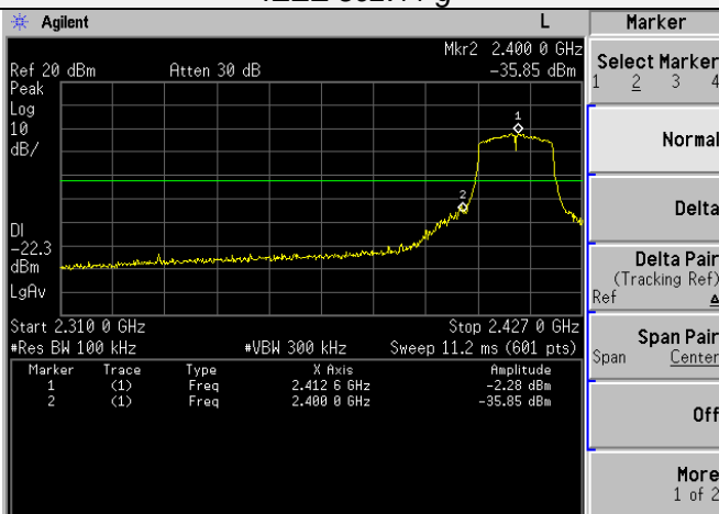
IEEE 802.11 g
