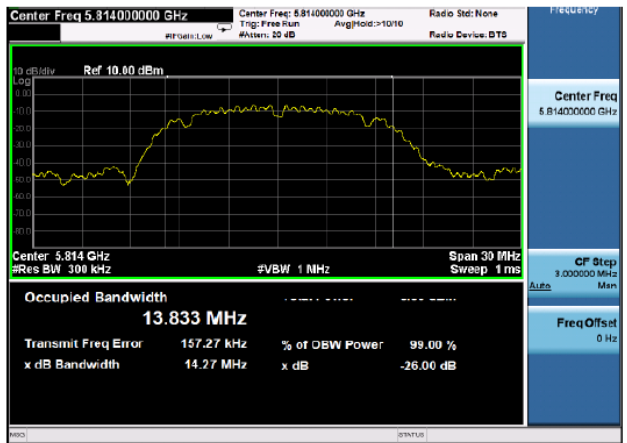
5814MHz-ANTA
