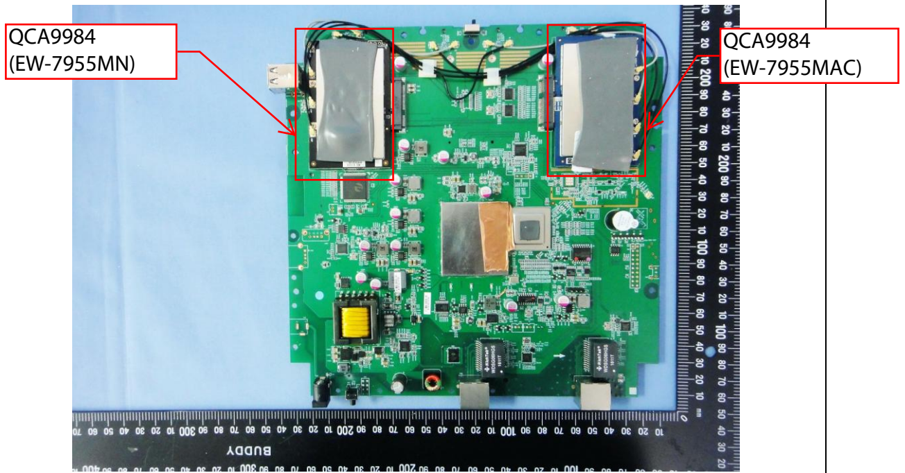
EUT Photo 20 )
