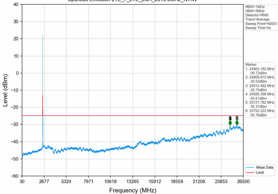
Spurious Emission LTE_7_LTE_LCH_2510.0MHz_NTNV
