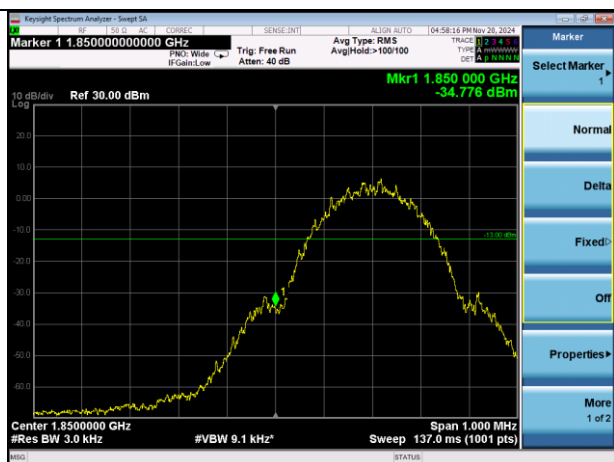
EGPRS1900L
