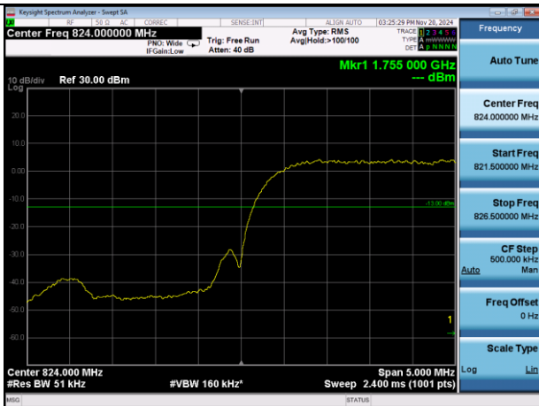
WCDMA B5/L
