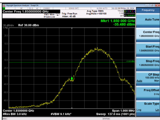
GPRS1900L
