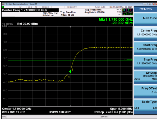
WCDMA B4/L
