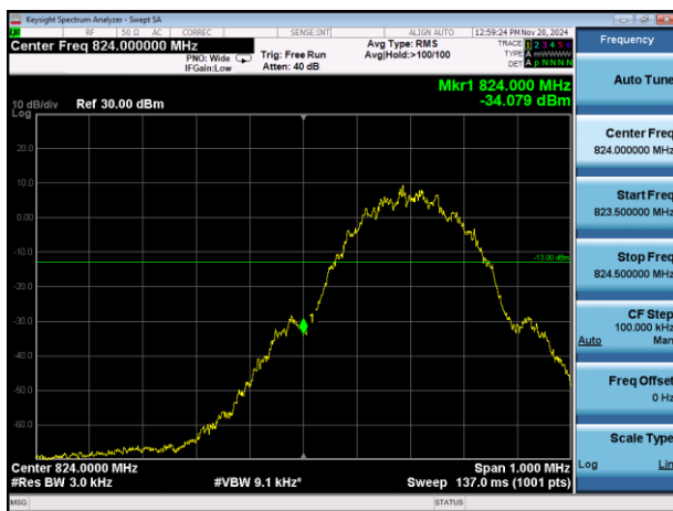
GPRS850\L
