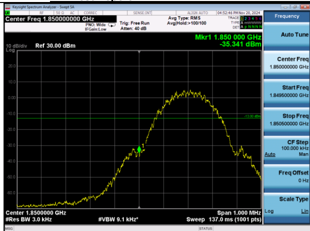
GSM1900L
