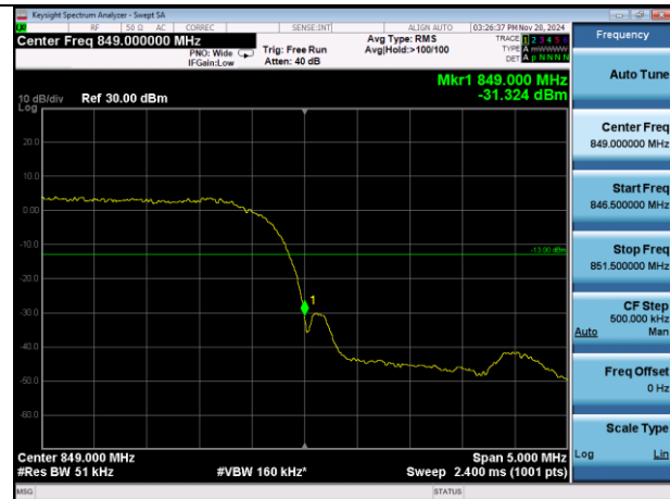
WCDMA B5/H
