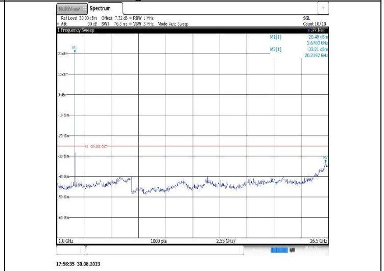
Band41-20MHz-QPSK-39750-1RB#0-Range2:1000~26500MHz
