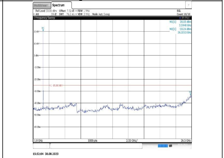
Band38-20MHz-QPSK-38150-1RB#0-Range2:1000~26500MHz
