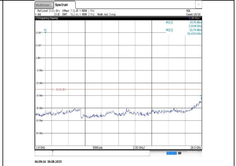
Band41-5MHz-QPSK-41565-1RB#0-Range2:1000~26500MHz
