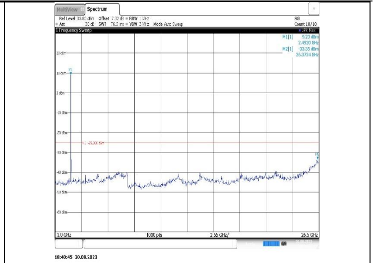
Band41-20MHz-QPSK-40620-1RB#0-Range2:1000~26500MHz
