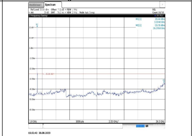
Band38-20MHz-16QAM-37850-1RB#0-Range2:1000~26500MHz
