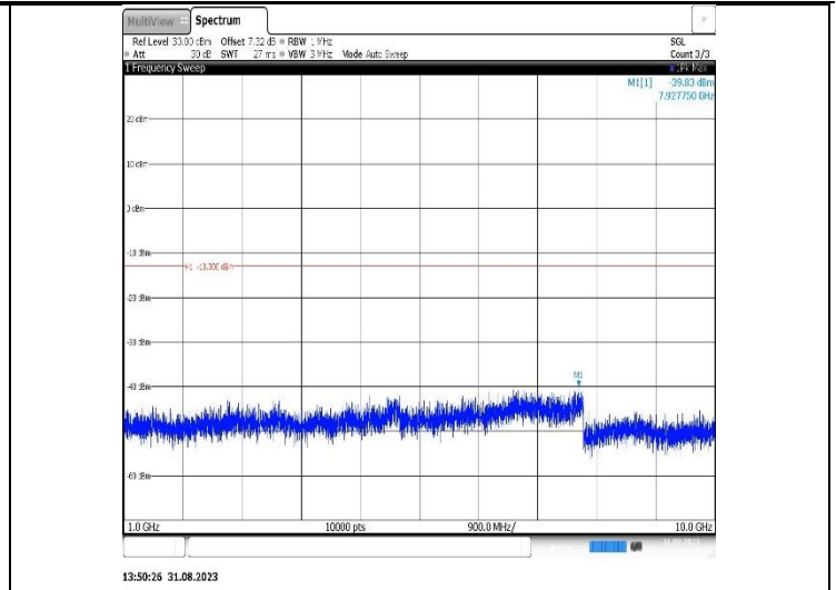
Band26(824-849)-15MHz-QPSK-26915-1RB#0-Range2:1000~10000MHz
