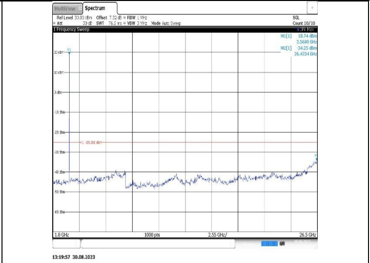
Band38-5MHz-QPSK-38000-1RB#0-Range2:1000~26500MHz
