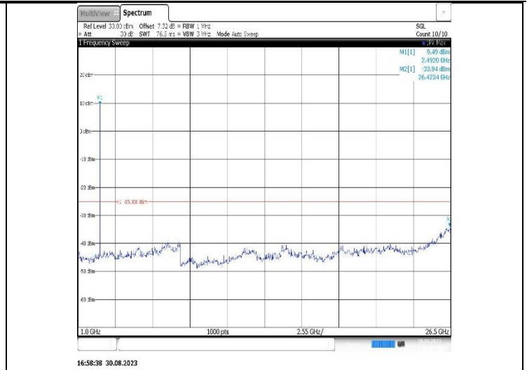
Band41-5MHz-QPSK-40620-1RB#0-Range2:1000~26500MHz
