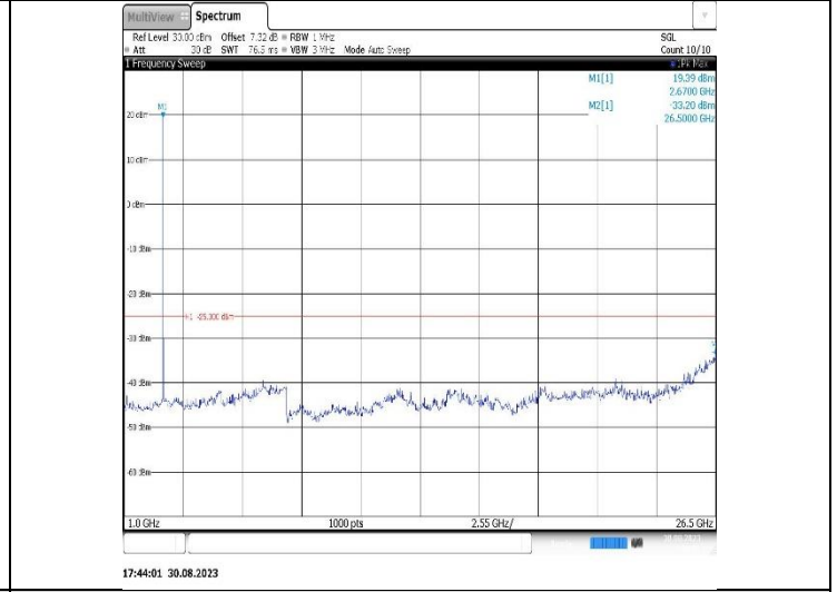
Band41-15MHz-QPSK-39725-1RB#0-Range2:1000~26500MHz
