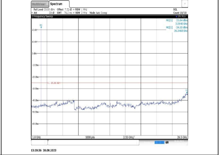
Band38-5MHz-QPSK-38225-1RB#0-Range2:1000~26500MHz
