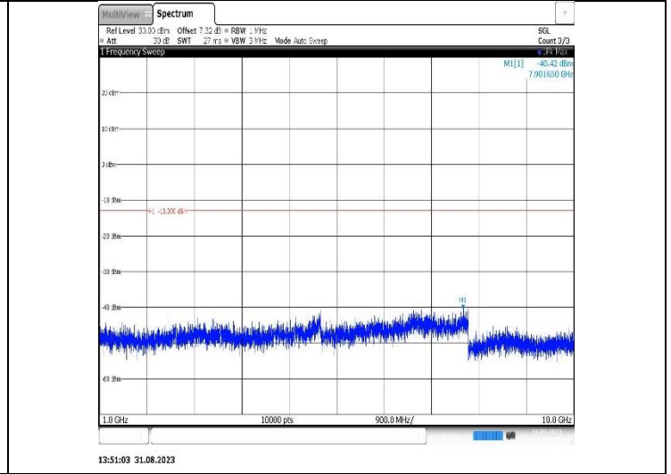
Band26(824-849)-15MHz-QPSK-26965-1RB#0-Range2:1000~10000MHz
