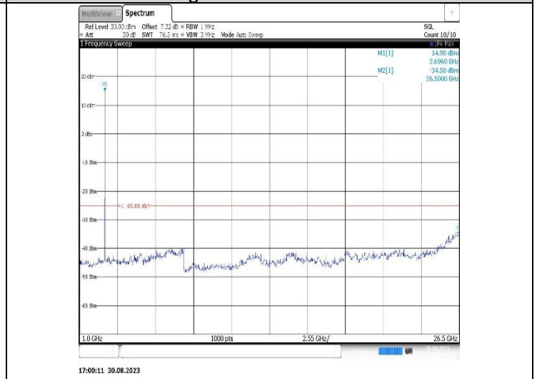
Band41-10MHz-QPSK-39700-1RB#0-Range2:1000~26500MHz
