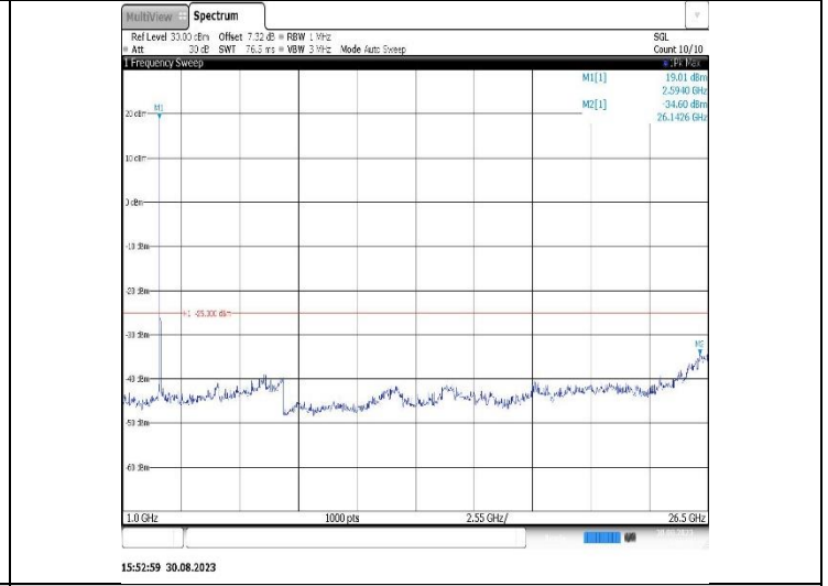
Band41-5MHz-QPSK-39675-1RB#0-Range2:1000~26500MHz
