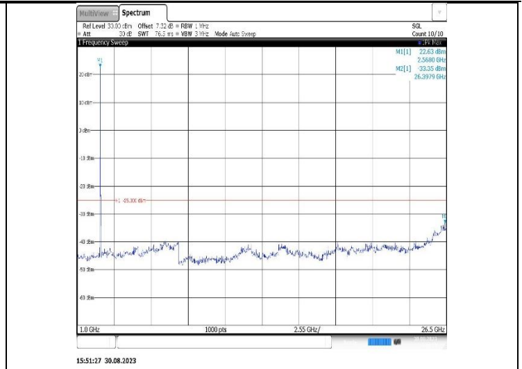
Band38-20MHz-QPSK-38000-1RB#0-Range2:1000~26500MHz
