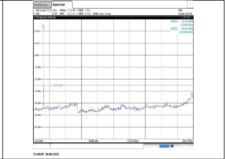
Band41-10MHz-QPSK-41540-1RB#0-Range2:1000~26500MHz
