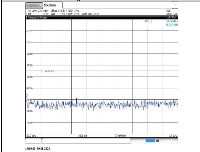
Band41-10MHz-QPSK-39700-1RB#0-Range1:30~1000MHz
