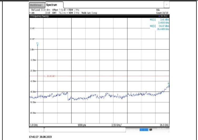
Band41-10MHz-QPSK-40620-1RB#0-Range2:1000~26500MHz
