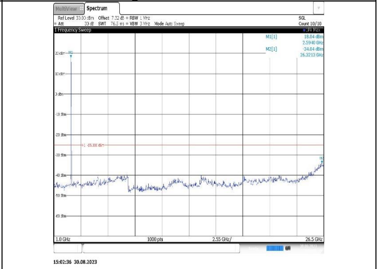
Band38-20MHz-QPSK-37850-1RB#0-Range2:1000~26500MHz
