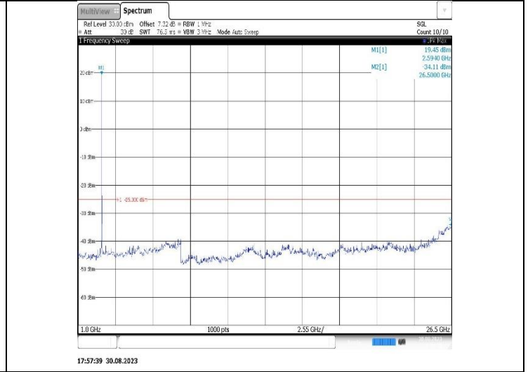
Band41-15MHz-QPSK-41515-1RB#0-Range2:1000~26500MHz
