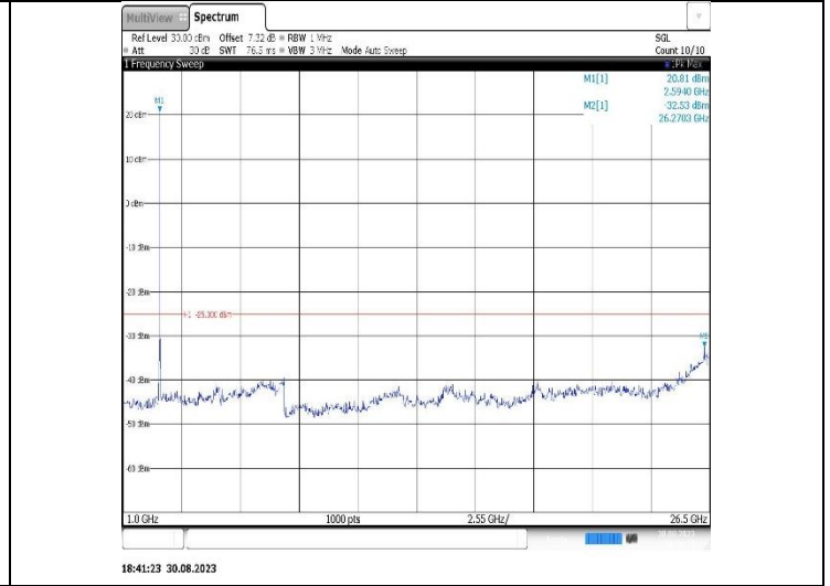
Band41-20MHz-QPSK-41490-1RB#0-Range2:1000~26500MHz
