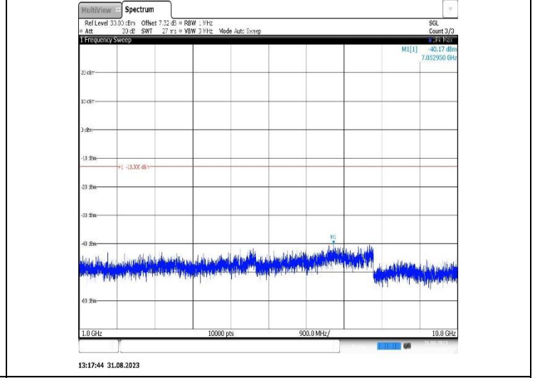
Band26(824-849)-5MHz-QPSK-27015-1RB#0-Range2:1000~10000MHz
