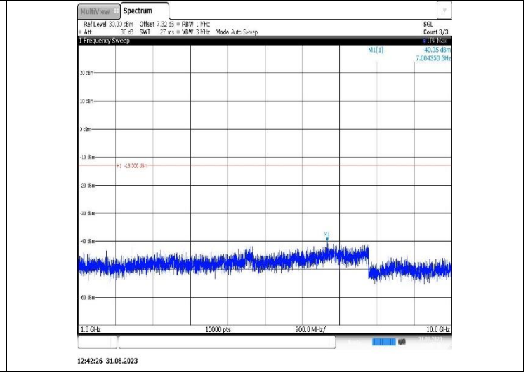
Band26(824-849)-3MHz-16QAM-27025-1RB#0-Range2:1000~10000MHz
