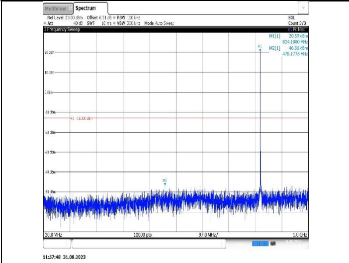
Band26(824-849)-1.4MHz-QPSK-26915-1RB#0-Range1:30~1000MHz
