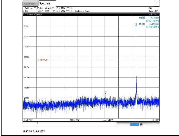
Band26(824-849)-5MHz-QPSK-27015-1RB#0-Range1:30~1000MHz
