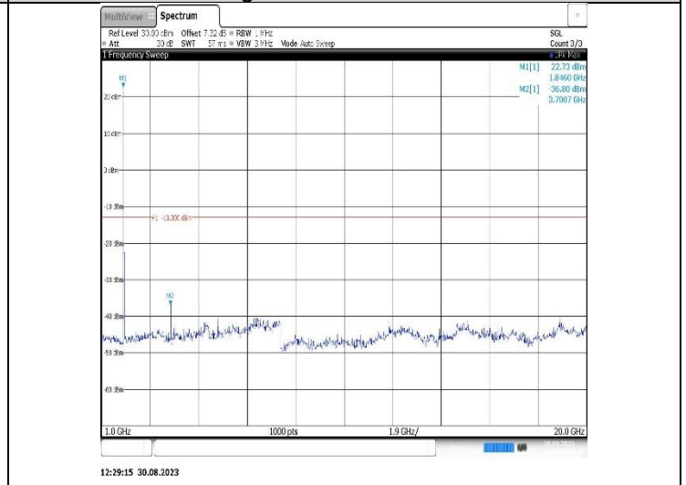
Band25-20MHz-16QAM-26365-1RB#0-Range2:1000~20000MHz
