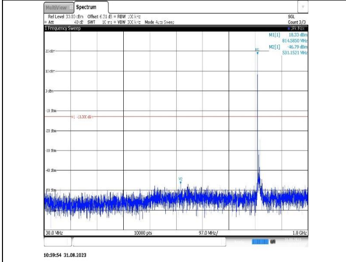
Band26(824-849)-1.4MHz-QPSK-26797-1RB#0-Range1:30~1000MHz
