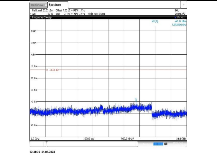
Band26(824-849)-3MHz-QPSK-26915-1RB#0-Range2:1000~10000MHz
