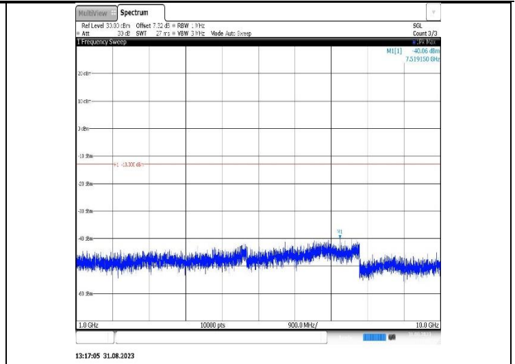
Band26(824-849)-5MHz-QPSK-26915-1RB#0-Range2:1000~10000MHz
