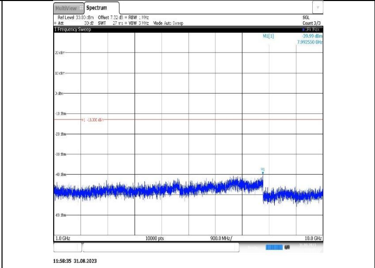
Band26(824-849)-1.4MHz-QPSK-27033-1RB#0-Range2:1000~10000MHz
