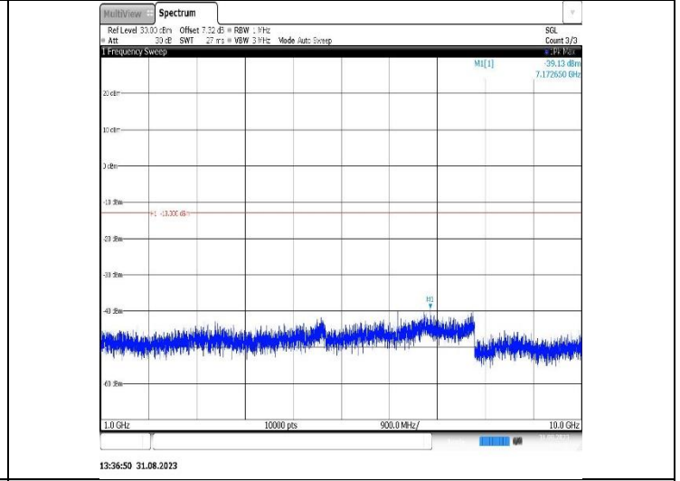
Band26(824-849)-15MHz-QPSK-26865-1RB#0-Range2:1000~10000MHz
