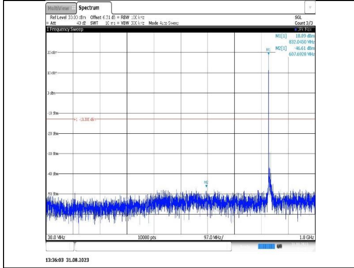
Band26(824-849)-10MHz-16QAM-26990-1RB#0-Range1:30~1000MHz
