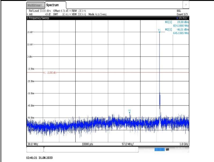
Band26(824-849)-3MHz-QPSK-26915-1RB#0-Range1:30~1000MHz
