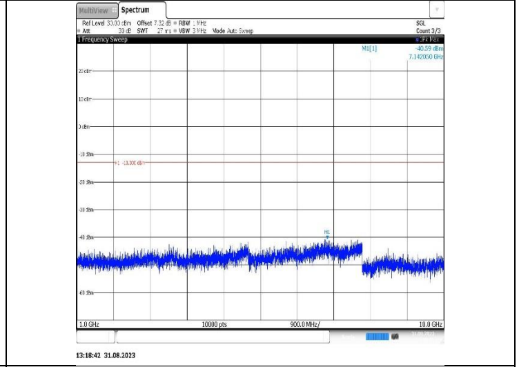
Band26(824-849)-10MHz-QPSK-26840-1RB#0-Range2:1000~10000MHz
