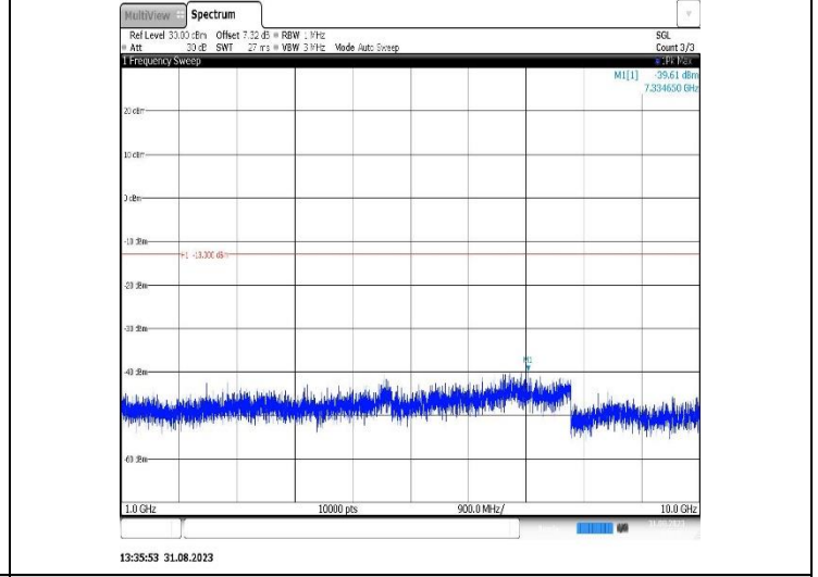
Band26(824-849)-10MHz-QPSK-26990-1RB#0-Range2:1000~10000MHz
