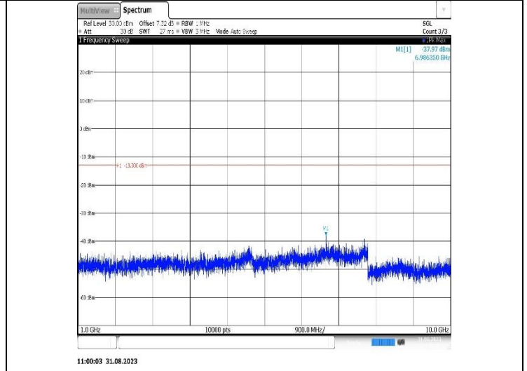
Band26(824-849)-1.4MHz-QPSK-26797-1RB#0-Range2:1000~10000MHz
