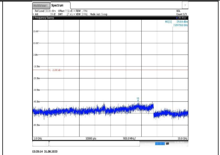
Band26(824-849)-10MHz-QPSK-26915-1RB#0-Range2:1000~10000MHz
