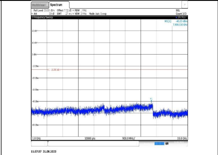
Band26(824-849)-1.4MHz-QPSK-26915-1RB#0-Range2:1000~10000MHz
