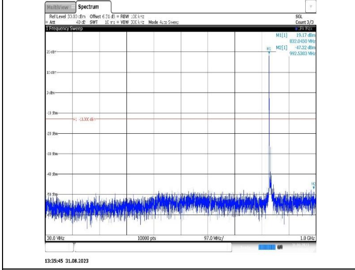
Band26(824-849)-10MHz-QPSK-26990-1RB#0-Range1:30~1000MHz
