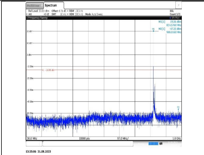
Band26(824-849)-10MHz-QPSK-26915-1RB#0-Range1:30~1000MHz
