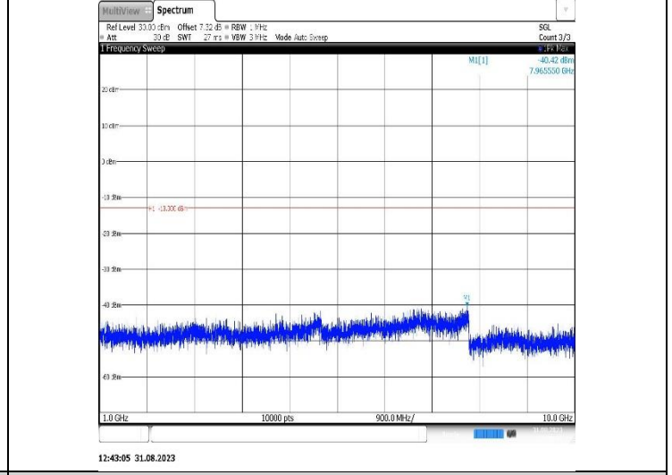
Band26(824-849)-5MHz-QPSK-26815-1RB#0-Range2:1000~10000MHz
