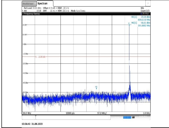
Band26(824-849)-15MHz-QPSK-26865-1RB#0-Range1:30~1000MHz
