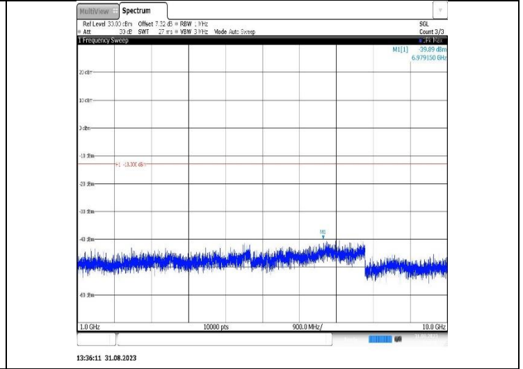
Band26(824-849)-10MHz-16QAM-26990-1RB#0-Range2:1000~10000MHz
