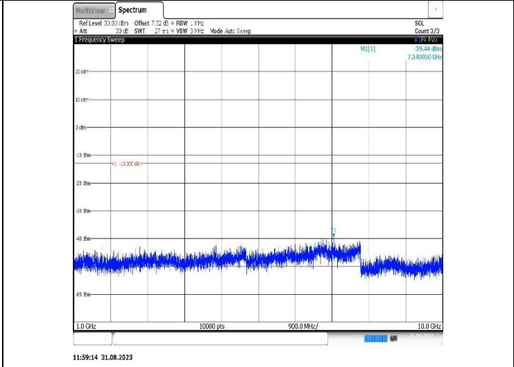
Band26(824-849)-1.4MHz-16QAM-26797-1RB#0-Range2:1000~10000MHz
