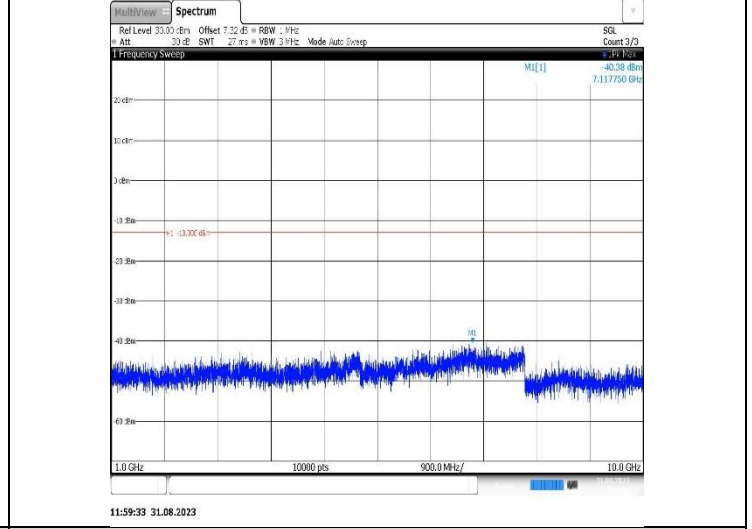
Band26(824-849)-3MHz-QPSK-26805-1RB#0-Range2:1000~10000MHz
