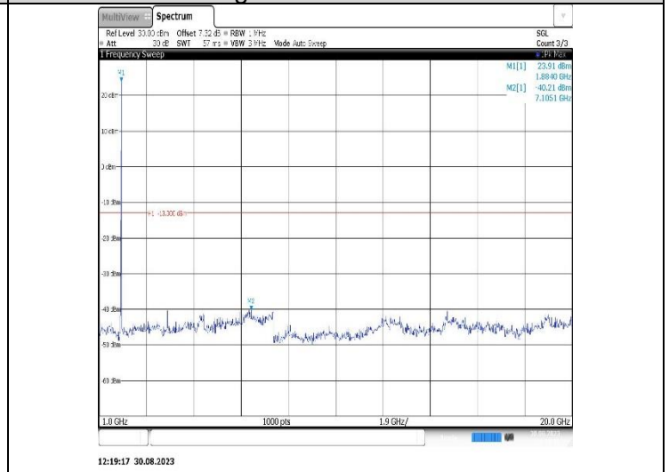
Band25-15MHz-QPSK-26615-1RB#0-Range2:1000~20000MHz
