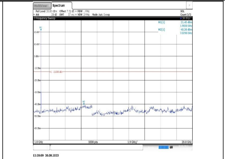
Band25-20MHz-QPSK-26140-1RB#0-Range2:1000~20000MHz
