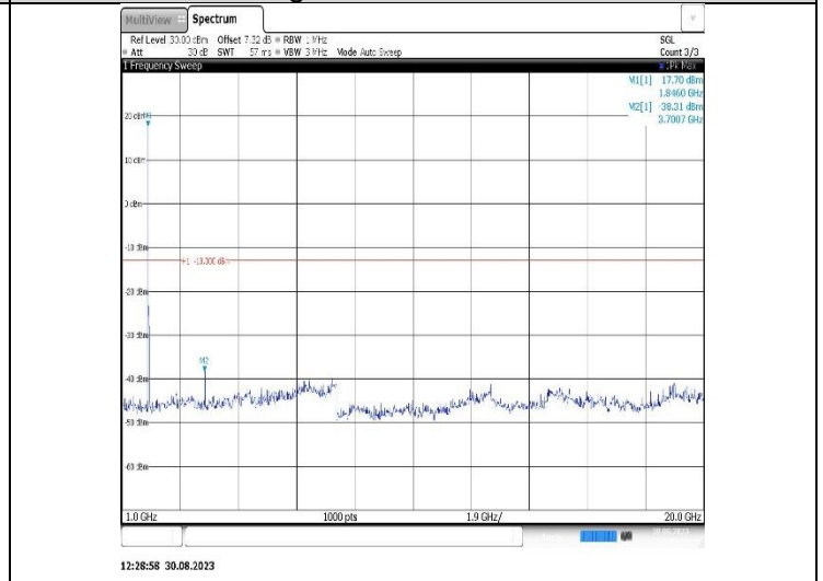
Band25-20MHz-QPSK-26365-1RB#0-Range2:1000~20000MHz
