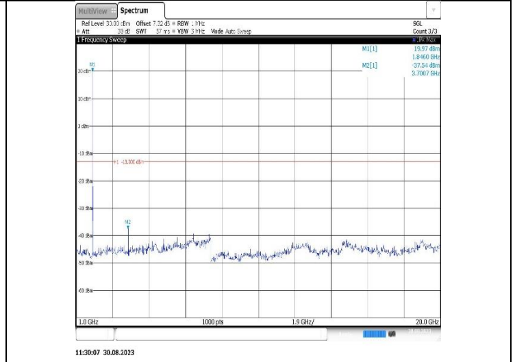
Band25-5MHz-QPSK-26365-1RB#0-Range2:1000~20000MHz
