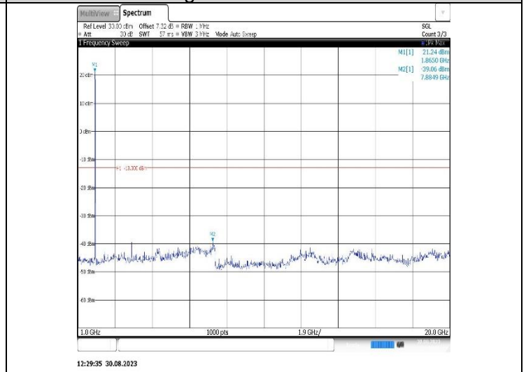
Band25-20MHz-QPSK-26590-1RB#0-Range2:1000~20000MHz
