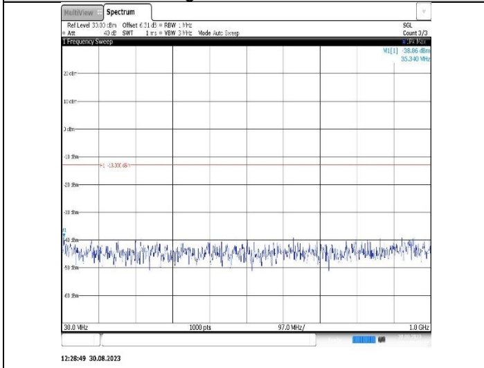
Band25-20MHz-QPSK-26365-1RB#0-Range1:30~1000MHz
