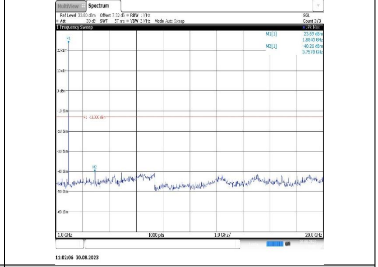
Band25-3MHz-QPSK-26675-1RB#0-Range2:1000~20000MHz
