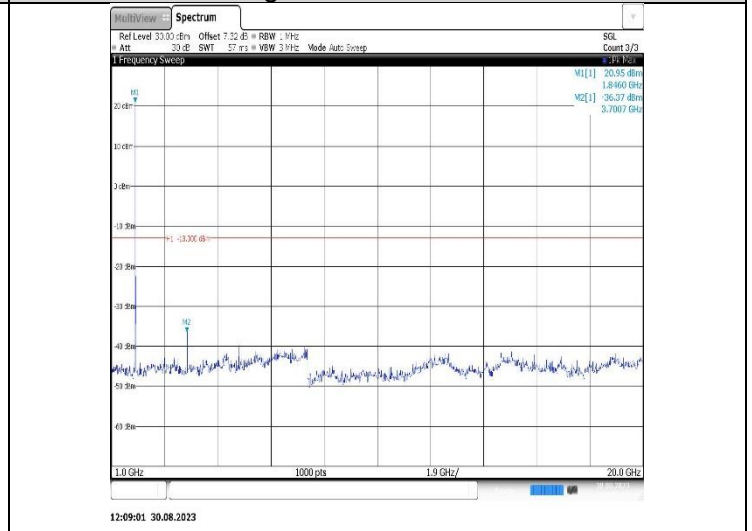
Band25-10MHz-QPSK-26365-1RB#0-Range2:1000~20000MHz
