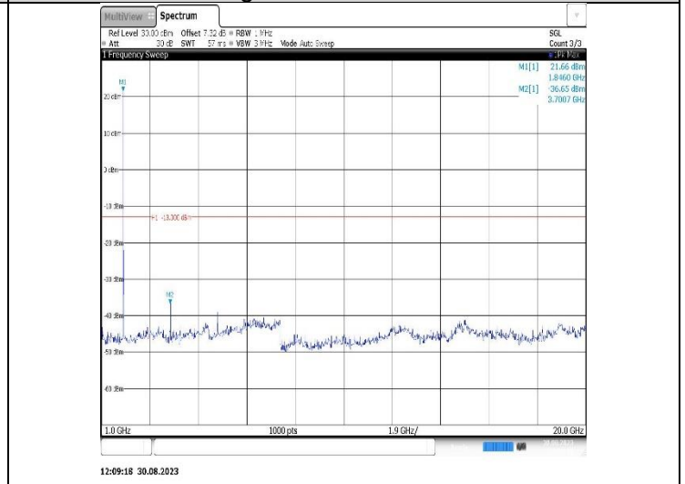
Band25-10MHz-16QAM-26365-1RB#0-Range2:1000~20000MHz
