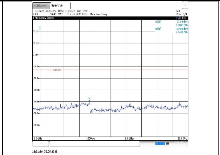
Band25-10MHz-QPSK-26090-1RB#0-Range2:1000~20000MHz
