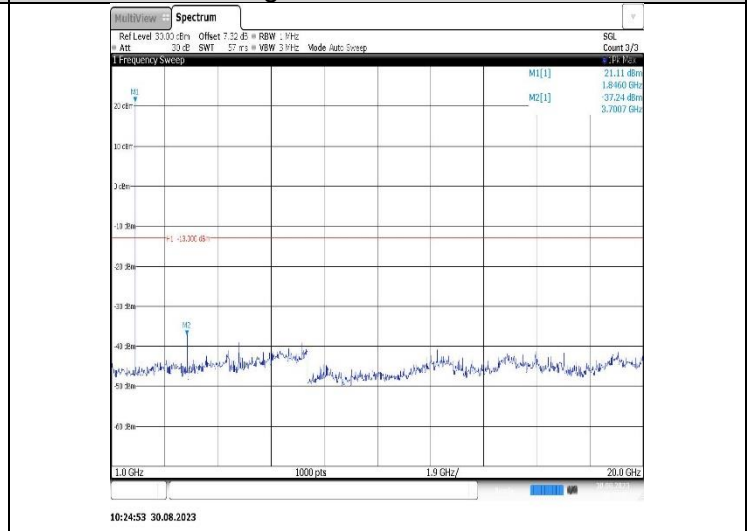
Band25-1.4MHz-QPSK-26365-1RB#0-Range2:1000~20000MHz
