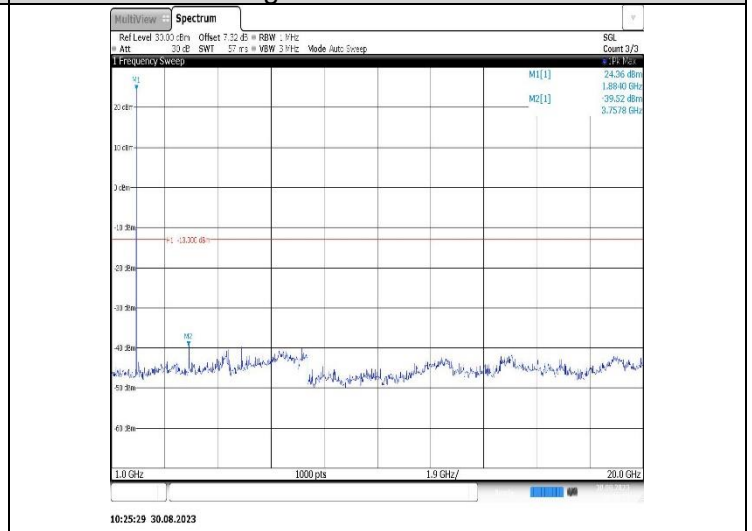
Band25-1.4MHz-QPSK-26683-1RB#0-Range2:1000~20000MHz
