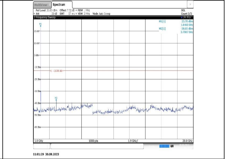
Band25-3MHz-QPSK-26365-1RB#0-Range2:1000~20000MHz
