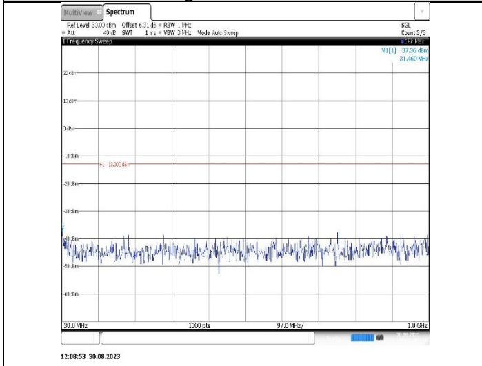
Band25-10MHz-QPSK-26365-1RB#0-Range1:30~1000MHz
