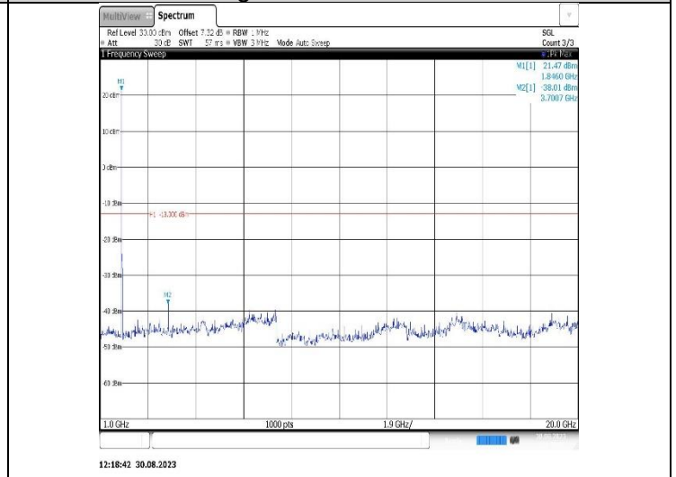
Band25-15MHz-QPSK-26365-1RB#0-Range2:1000~20000MHz
