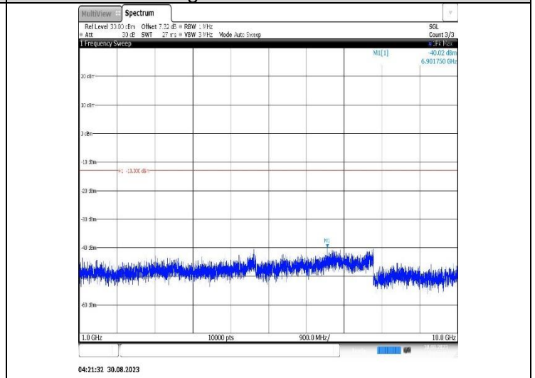
Band12-5MHz-QPSK-23155-1RB#0- Range2:1000~10000MHz
