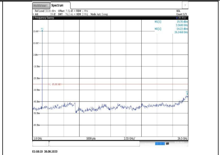
Band7-10MHz-QPSK-20800-1RB#0-Range2:1000~26500MHz
