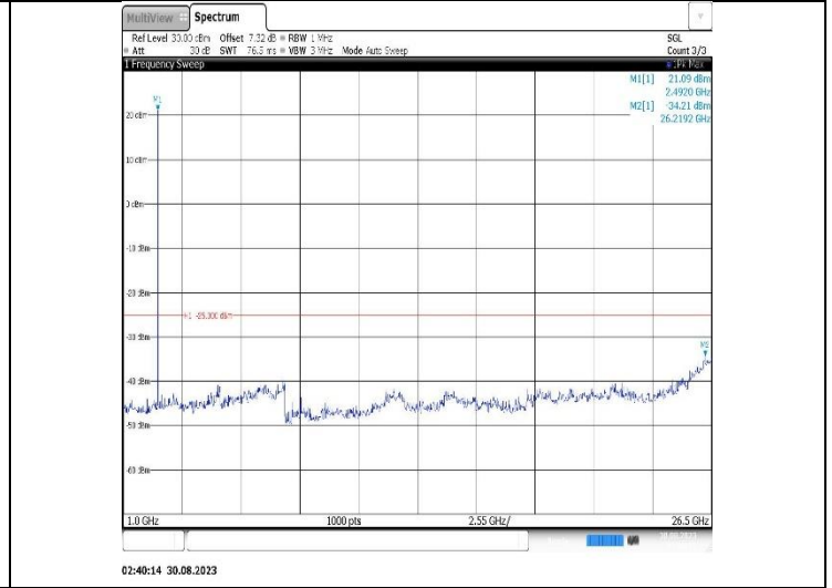
Band7-10MHz-QPSK-21100-1RB#0-Range2:1000~26500MHz
