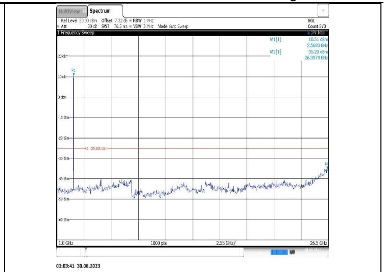
Band7-20MHz-QPSK-20850-1RB#0-Range2:1000~26500MHz
