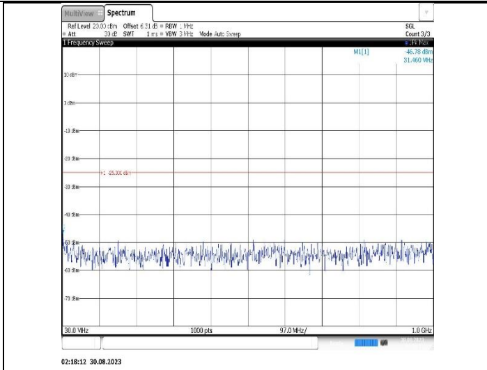
Band7-10MHz-QPSK-20800-1RB#0-Range1:30~1000MHz
