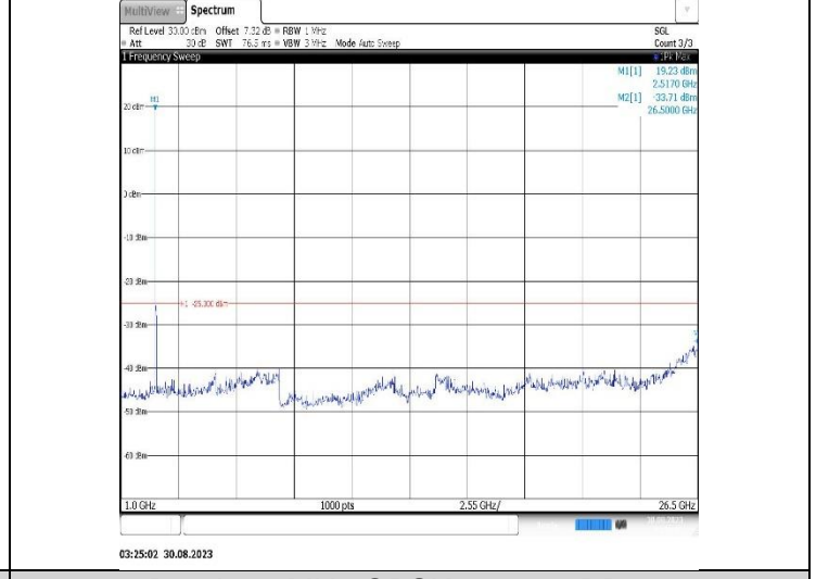
Band7-20MHz-QPSK-21350-1RB#0-Range2:1000~26500MHz
