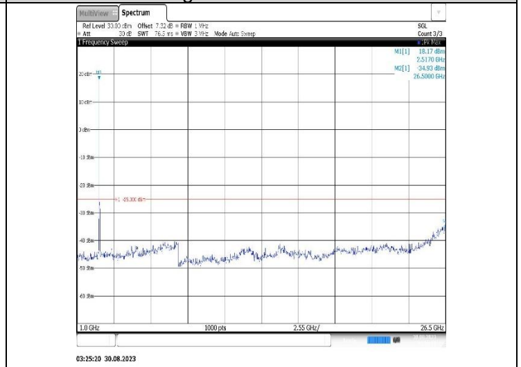
Band7-20MHz-16QAM-21350-1RB#0-Range2:1000~26500MHz
