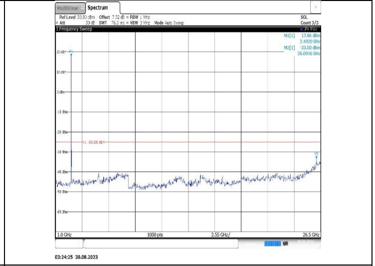
Band7-20MHz-QPSK-21100-1RB#0-Range2:1000~26500MHz
