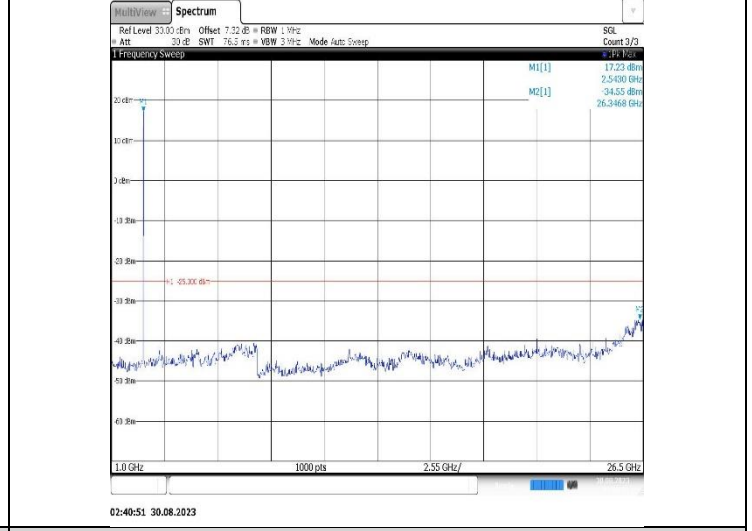
Band7-10MHz-QPSK-21400-1RB#0-Range2:1000~26500MHz
