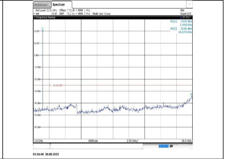
Band7-5MHz-QPSK-21100-1RB#0-Range2:1000~26500MHz
