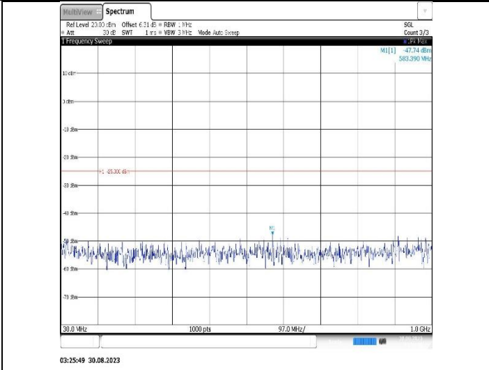
Band12-1.4MHz-QPSK-23017-1RB#0-Range1:30~1000MHz
