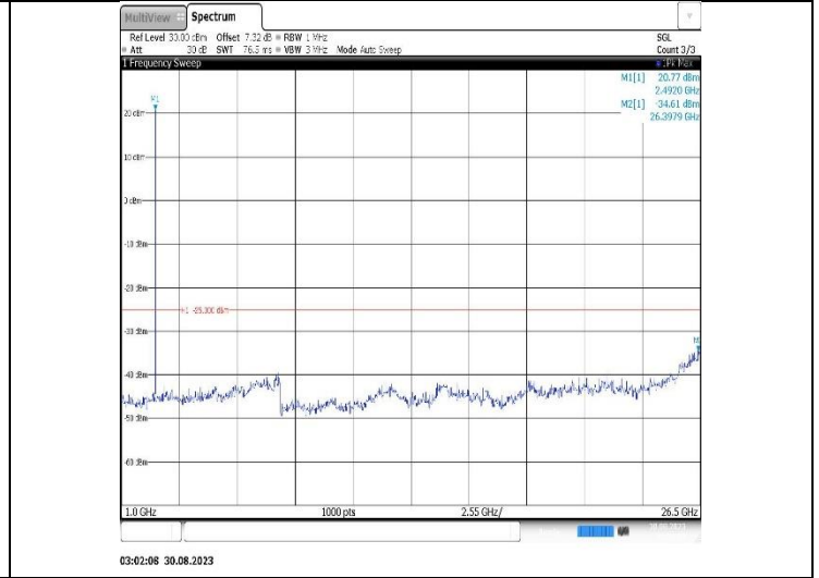
Band7-15MHz-QPSK-21100-1RB#0- Range2:1000~26500MHz
