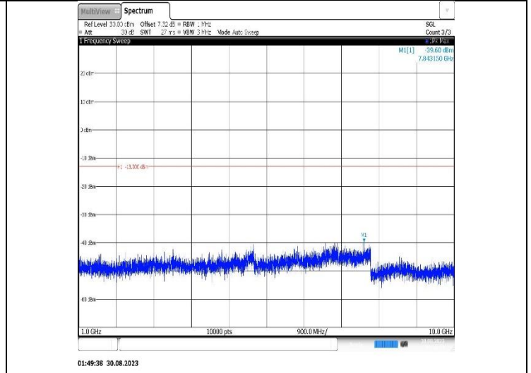
Band5-10MHz-QPSK-20525-1RB#0- Range2:1000~10000MHz
