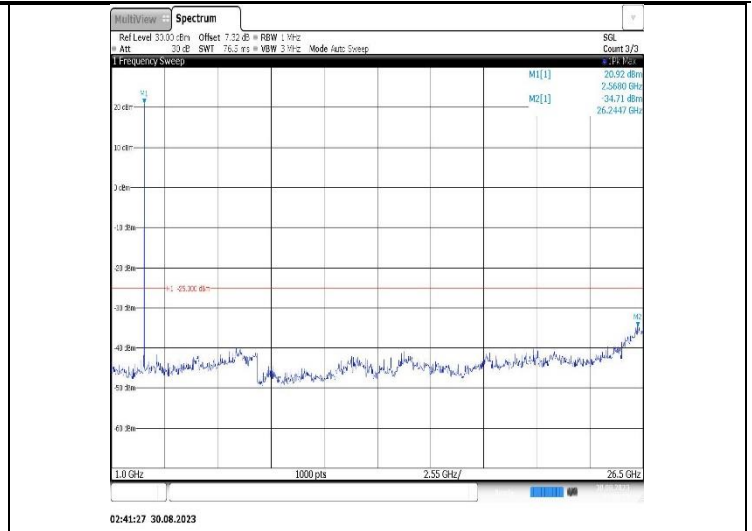
Band7-10MHz-16QAM-20800-1RB#0-Range2:1000~26500MHz
