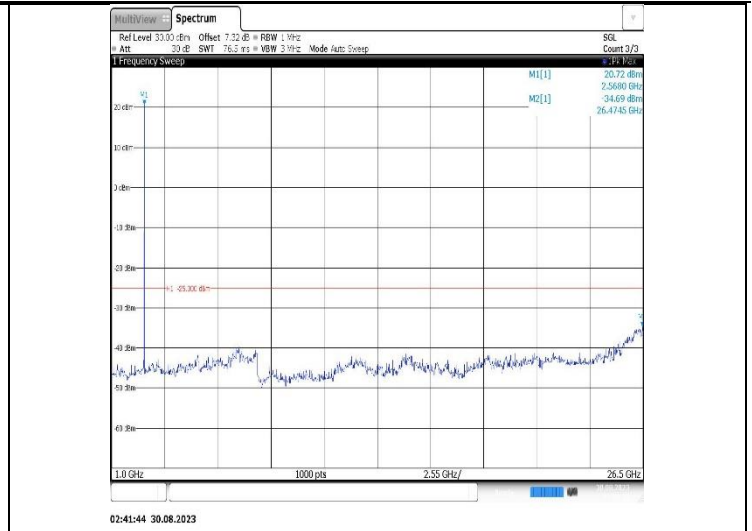
Band7-15MHz-QPSK-20825-1RB#0- Range2:1000~26500MHz
