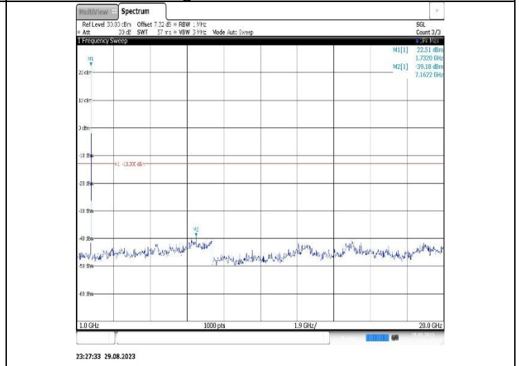
Band4-10MHz-QPSK-20350-1RB#0- Range2:1000~20000MHz
