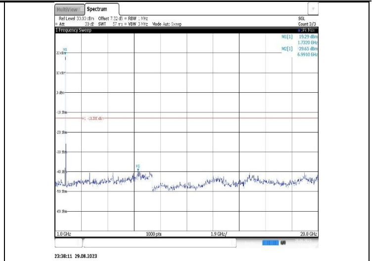
Band4-20MHz-QPSK-20050-1RB#0- Range2:1000~20000MHz
