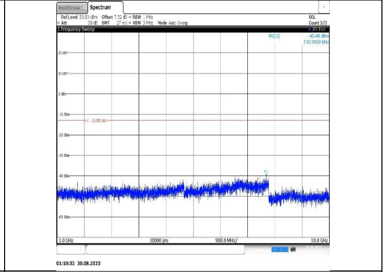
Band5-3MHz-QPSK-20635-1RB#0-Range2:1000~10000MHz
