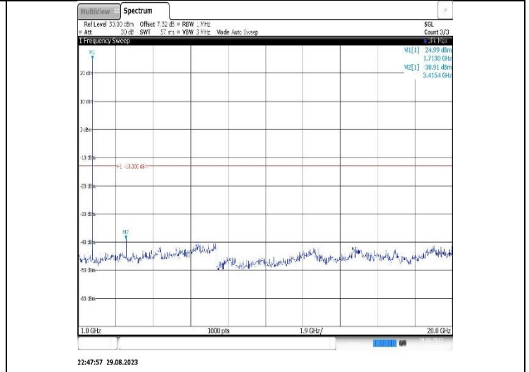
Band4-5MHz-QPSK-20175-1RB#0-Range2:1000~20000MHz
