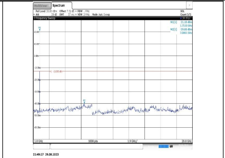
Band4-10MHz-QPSK-20000-1RB#0- Range2:1000~20000MHz
