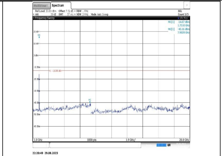
Band4-5MHz-QPSK-19975-1RB#0-Range2:1000~20000MHz
