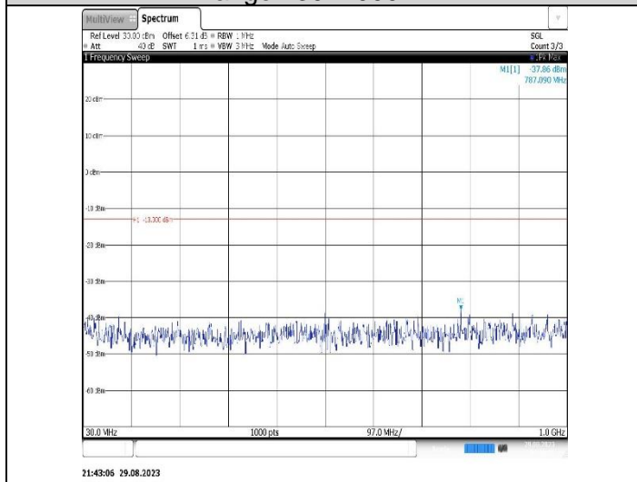
Band4-1.4MHz-QPSK-20393-1RB#0- Range1:30~1000MHz
