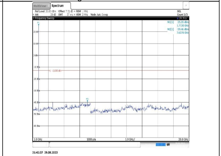
Band4-1.4MHz-QPSK-20175-1RB#0- Range2:1000~20000MHz
