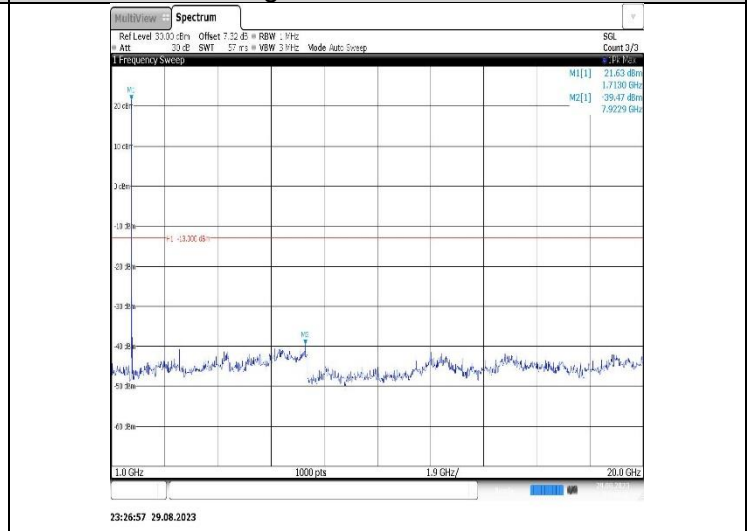
Band4-10MHz-QPSK-20175-1RB#0- Range2:1000~20000MHz
