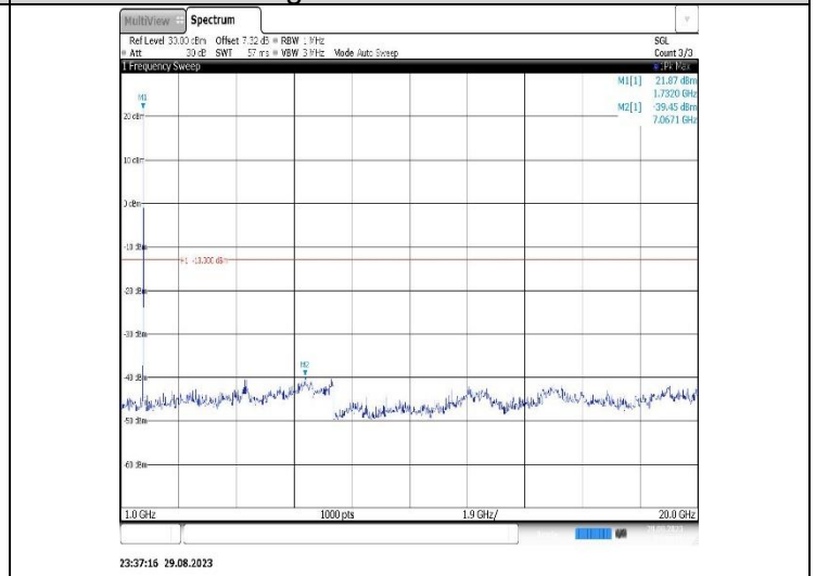
Band4-15MHz-QPSK-20325-1RB#0- Range2:1000~20000MHz
