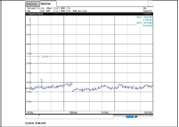
Band4-3MHz-QPSK-20175-1RB#0-Range2:1000~20000MHz
