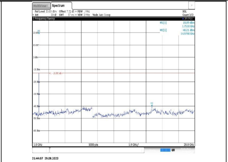
Band4-3MHz-QPSK-19965-1RB#0-Range2:1000~20000MHz
