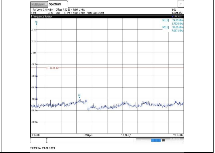
Band4-3MHz-QPSK-20385-1RB#0-Range2:1000~20000MHz
