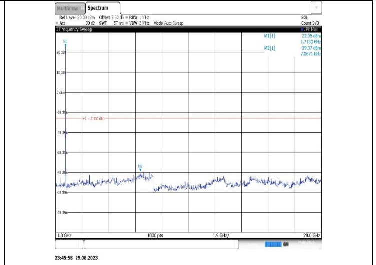
Band4-20MHz-QPSK-20175-1RB#0- Range2:1000~20000MHz
