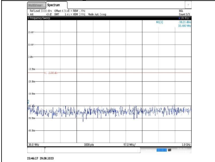
Band4-20MHz-QPSK-20300-1RB#0- Range1:30~1000MHz
