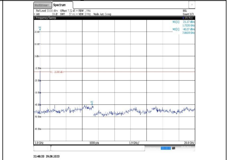
Band4-5MHz-QPSK-20375-1RB#0-Range2:1000~20000MHz
