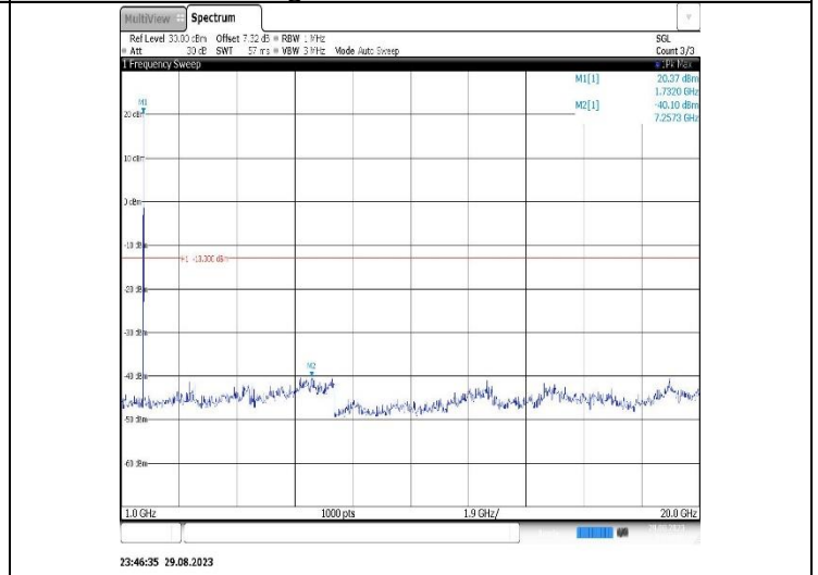
Band4-20MHz-QPSK-20300-1RB#0- Range2:1000~20000MHz
