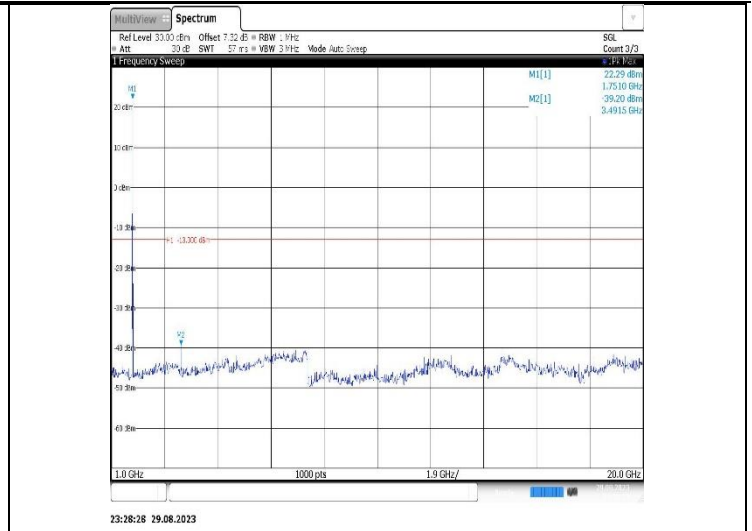
Band4-15MHz-QPSK-20025-1RB#0- Range2:1000~20000MHz
