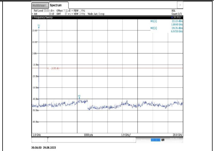
Band4-1.4MHz-QPSK-19957-1RB#0- Range2:1000~20000MHz
