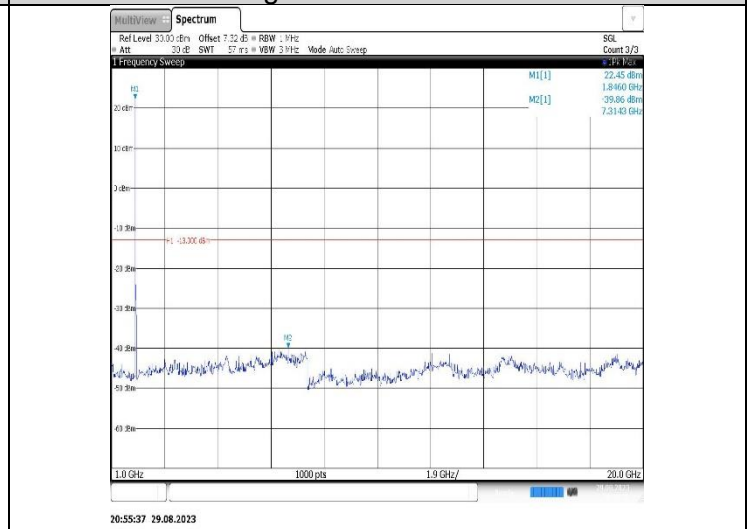
Band2-20MHz-16QAM-18900-1RB#0-Range2:1000~20000MHz
