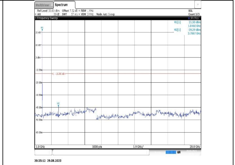
Band2-10MHz-QPSK-18900-1RB#0-Range2:1000~20000MHz
