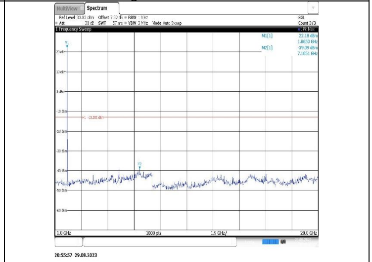
Band2-20MHz-QPSK-19100-1RB#0- Range2:1000~20000MHz
