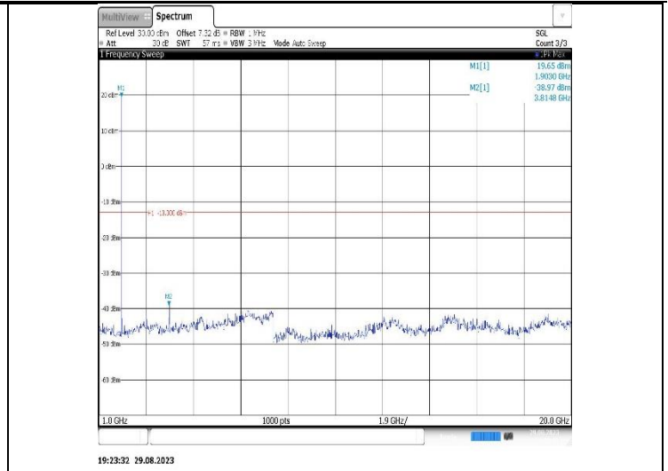
Band2-3MHz-QPSK-18615-1RB#0-Range2:1000~20000MHz
