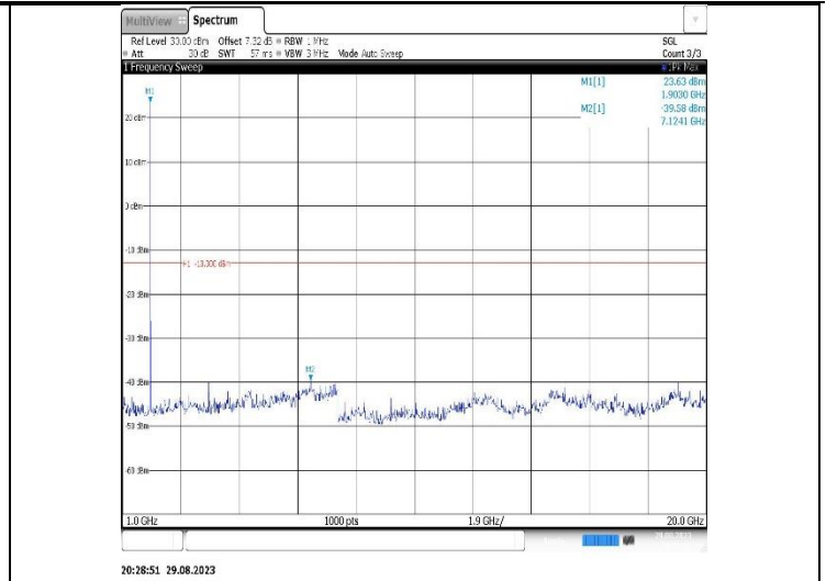
Band2-10MHz-QPSK-18650-1RB#0-Range2:1000~20000MHz
