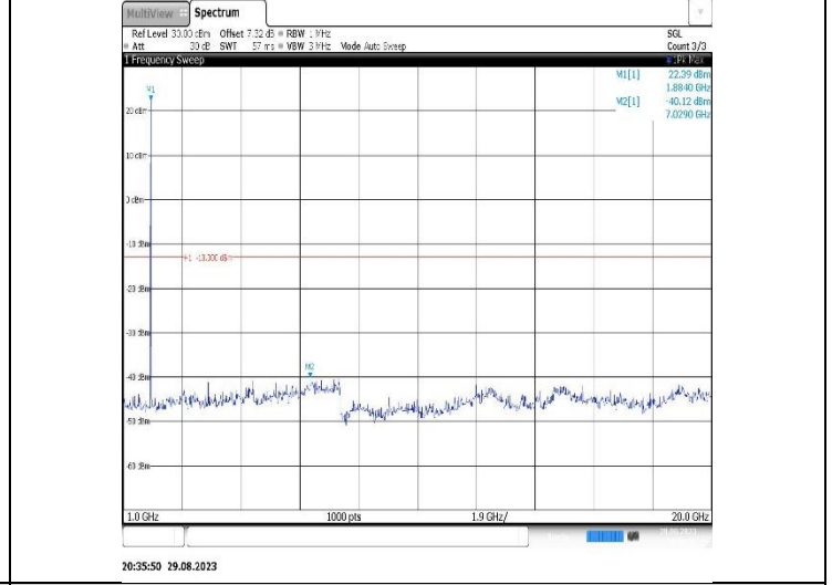
Band2-10MHz-QPSK-19150-1RB#0-Range2:1000~20000MHz
