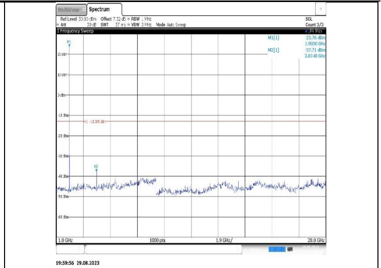
Band2-3MHz-16QAM-18615-1RB#0-Range2:1000~20000MHz
