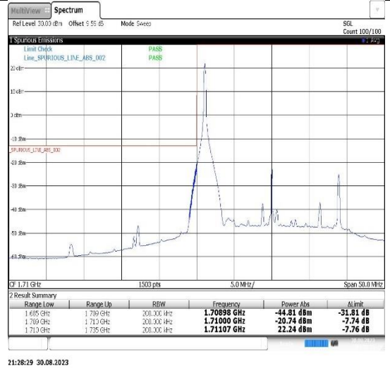
Band66-20MHz-QPSK-132572-1RB#99
