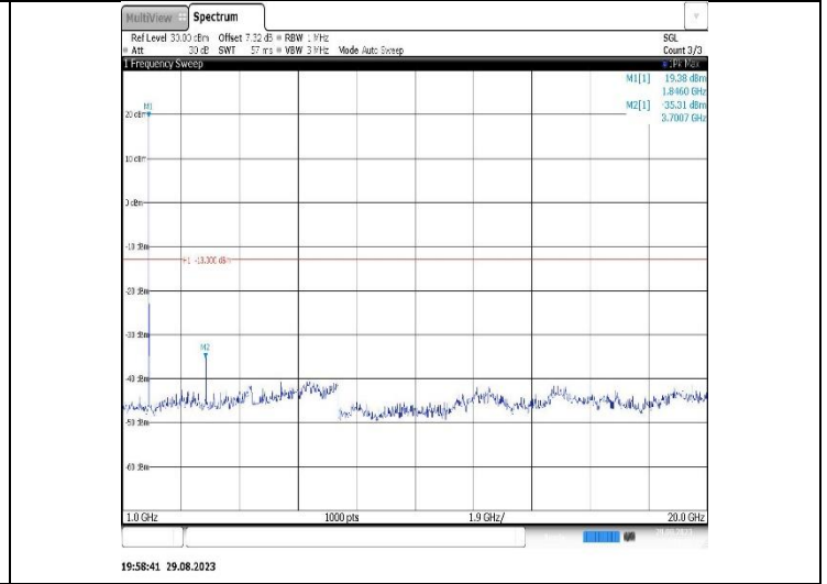
Band2-3MHz-QPSK-18900-1RB#0-Range2:1000~20000MHz
