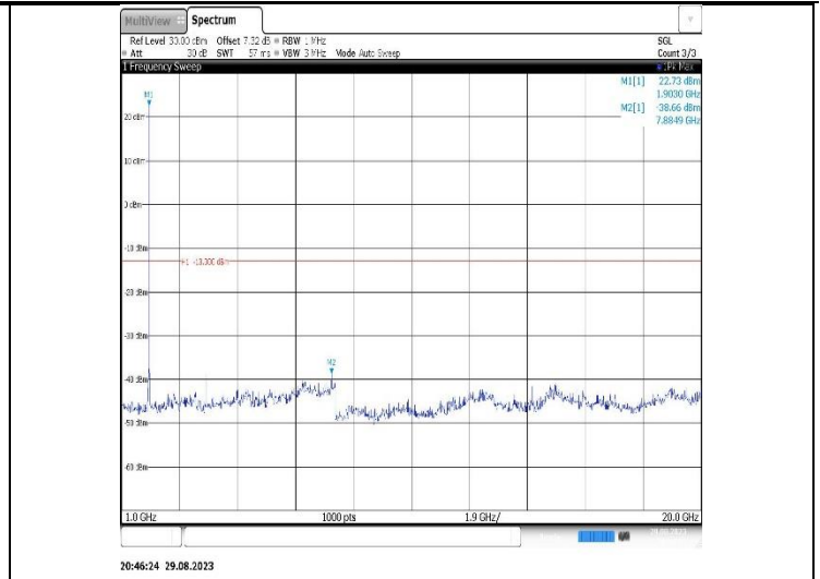
Band2-20MHz-QPSK-18700-1RB#0- Range2:1000~20000MHz
