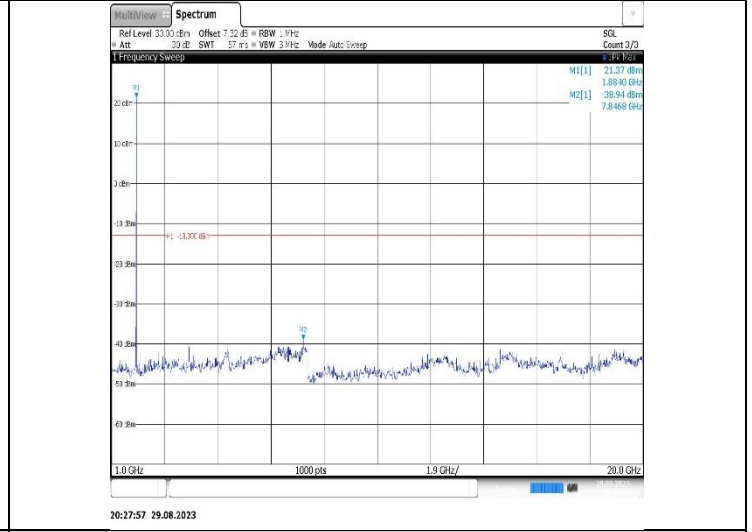
Band2-5MHz-QPSK-19175-1RB#0-Range2:1000~20000MHz
