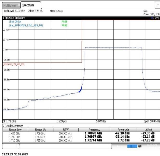
Band66-20MHz-QPSK-132572-100RB#0
