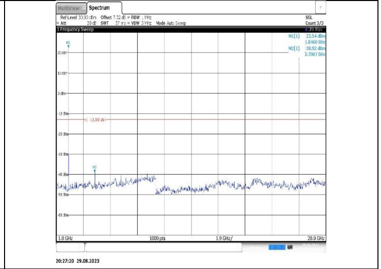
Band2-5MHz-QPSK-18900-1RB#0-Range2:1000~20000MHz
