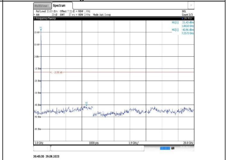
Band2-15MHz-QPSK-19125-1RB#0- Range2:1000~20000MHz
