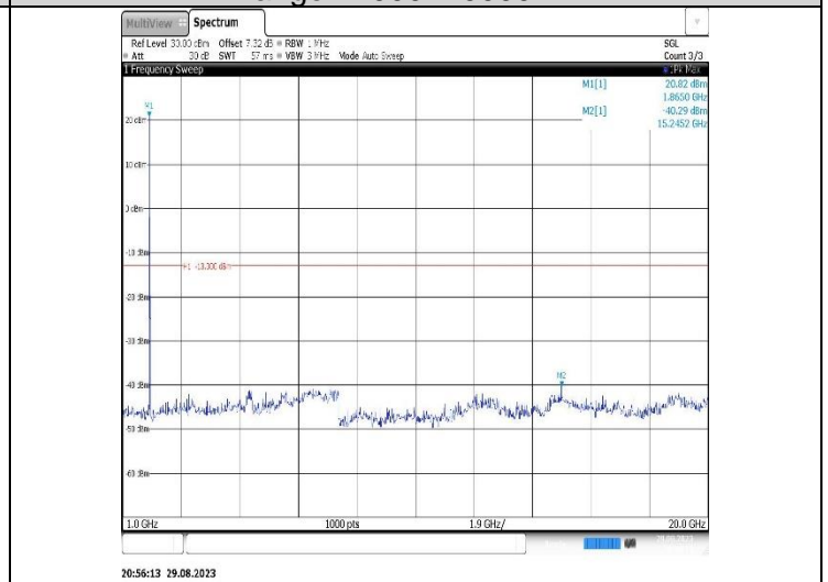
Band2-20MHz-16QAM-19100-1RB#0-Range2:1000~20000MHz
