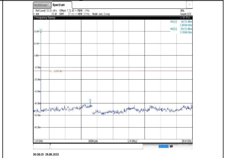
Band2-5MHz-16QAM-19175-1RB#0- Range2:1000~20000MHz
