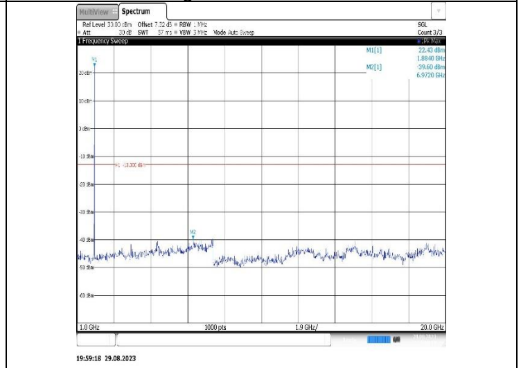
Band2-3MHz-QPSK-19185-1RB#0-Range2:1000~20000MHz
