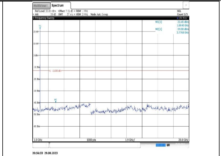
Band2-20MHz-16QAM-18700-1RB#0-Range2:1000~20000MHz
