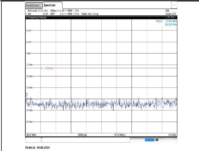
Band2-20MHz-QPSK-18700-1RB#0- Range1:30~1000MHz
