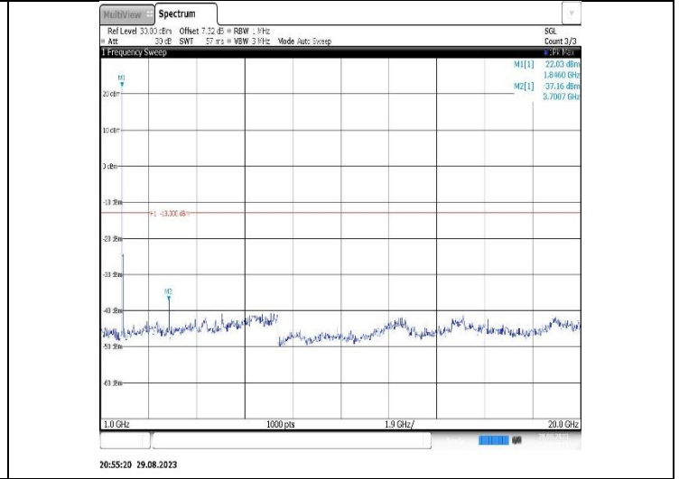
Band2-20MHz-QPSK-18900-1RB#0- Range2:1000~20000MHz
