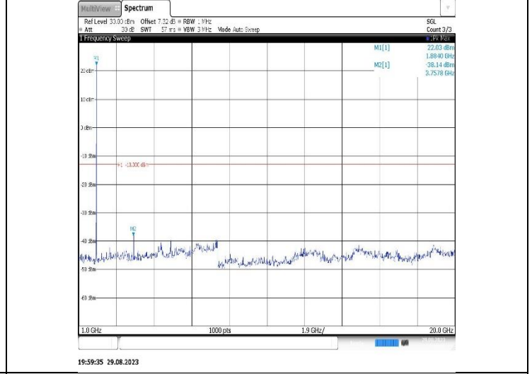
Band2-3MHz-16QAM-19185-1RB#0-Range2:1000~20000MHz
