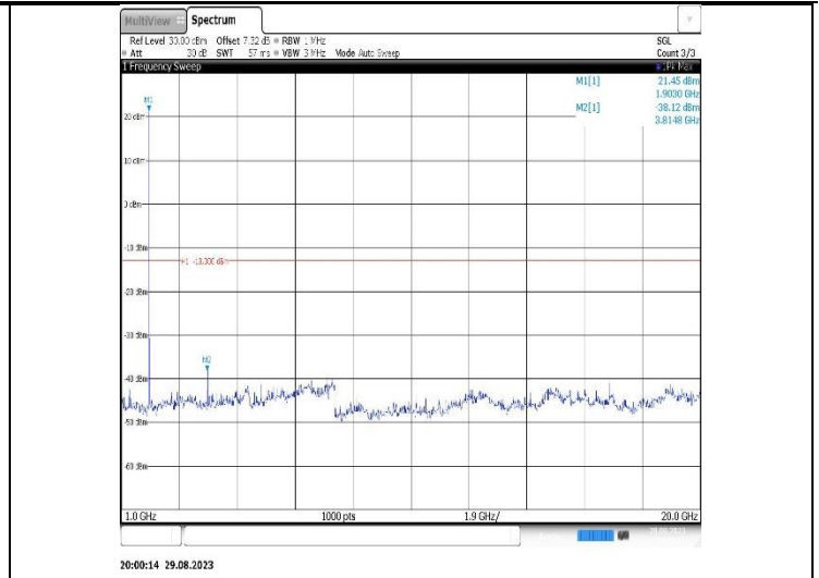
Band2-5MHz-QPSK-18625-1RB#0-Range2:1000~20000MHz
