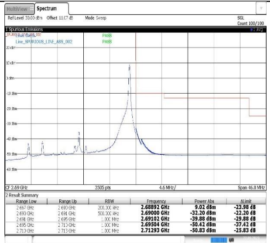
Band41-20MHz-QPSK-41490-1RB#99
