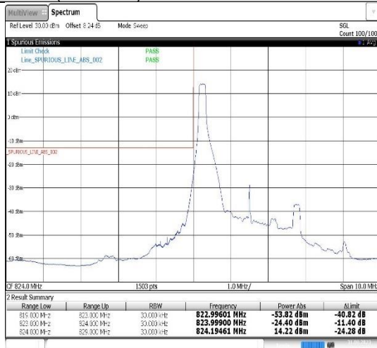
Band26(824-849)-3MHz-QPSK-26805-1RB#0
