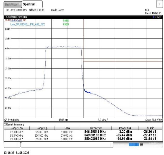
Band26(824-849)-10MHz-QPSK-26840-50RB#0
