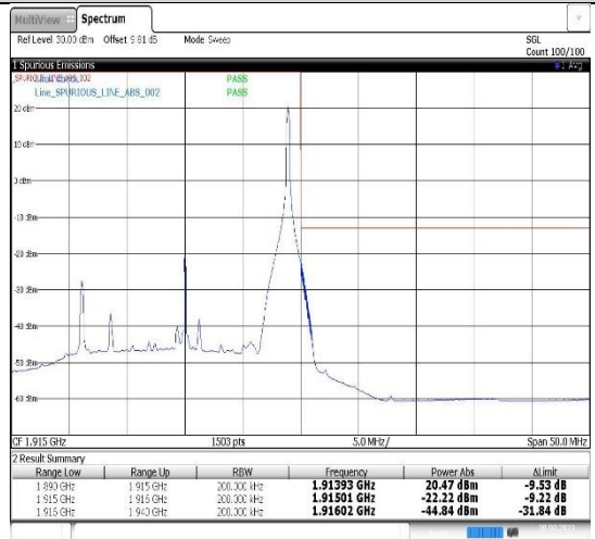
Band25-20MHz-16QAM-26590-1RB#99
