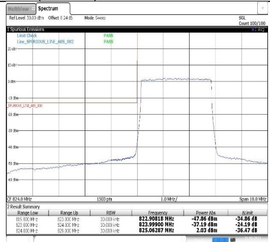
Band26(824-849)-3MHz-QPSK-26805-15RB#0
