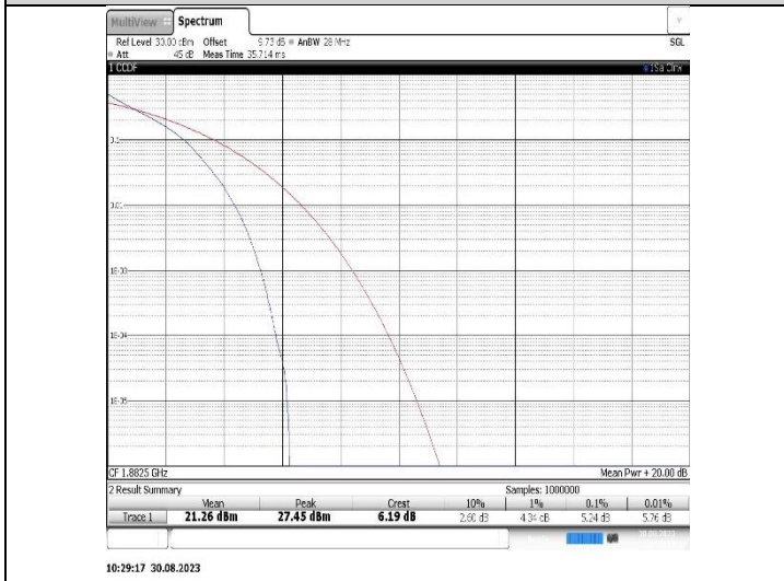
Band25-3MHz-QPSK-26365-15RB#0
