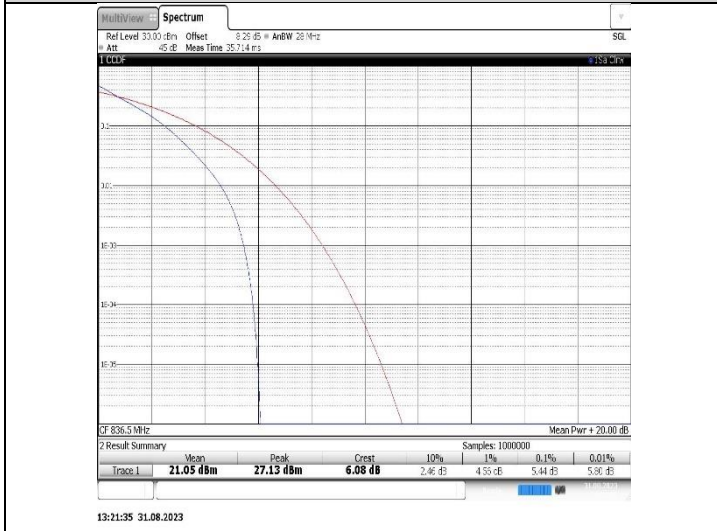
Band26(824-849)-10MHz-QPSK-26915-50RB#0
