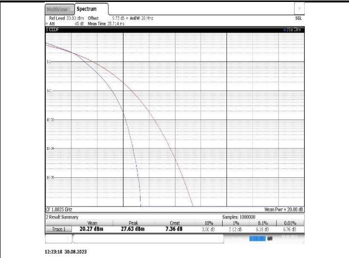
Band25-20MHz-16QAM-26365-100RB#0
