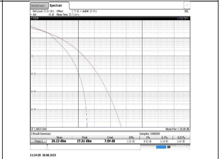
Band25-10MHz-16QAM-26365-50RB#0
