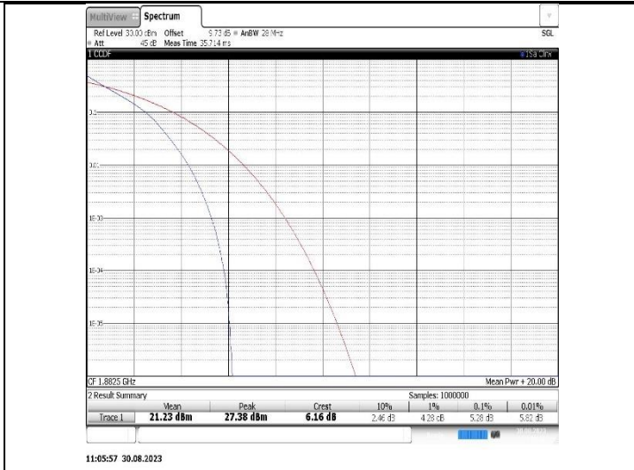
Band25-5MHz-QPSK-26365-25RB#0
