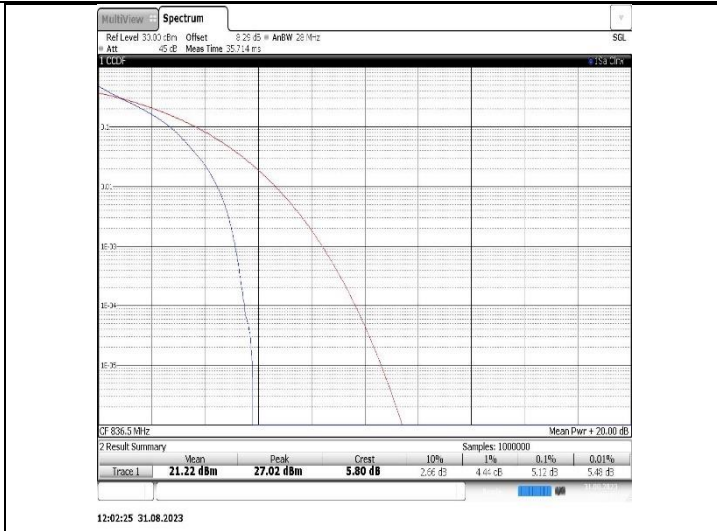
Band26(824-849)-3MHz-QPSK-26915-15RB#0
