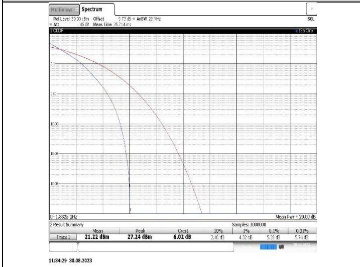
Band25-10MHz-QPSK-26365-50RB#0
