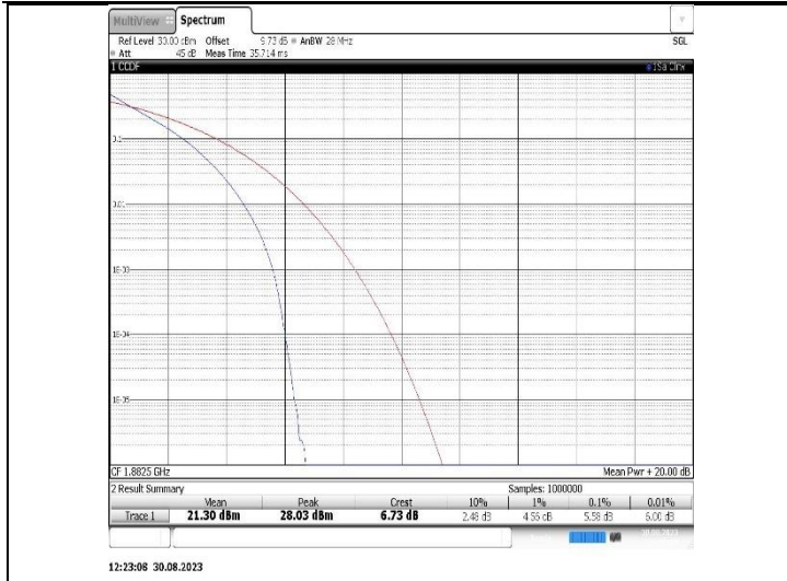
Band25-20MHz-QPSK-26365-100RB#0
