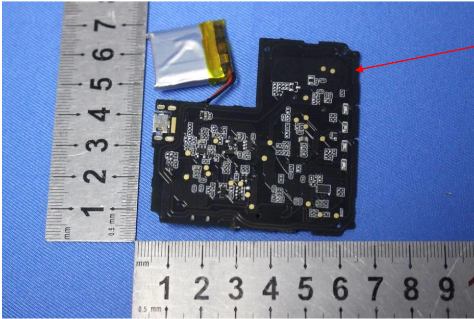
NFC antenna
