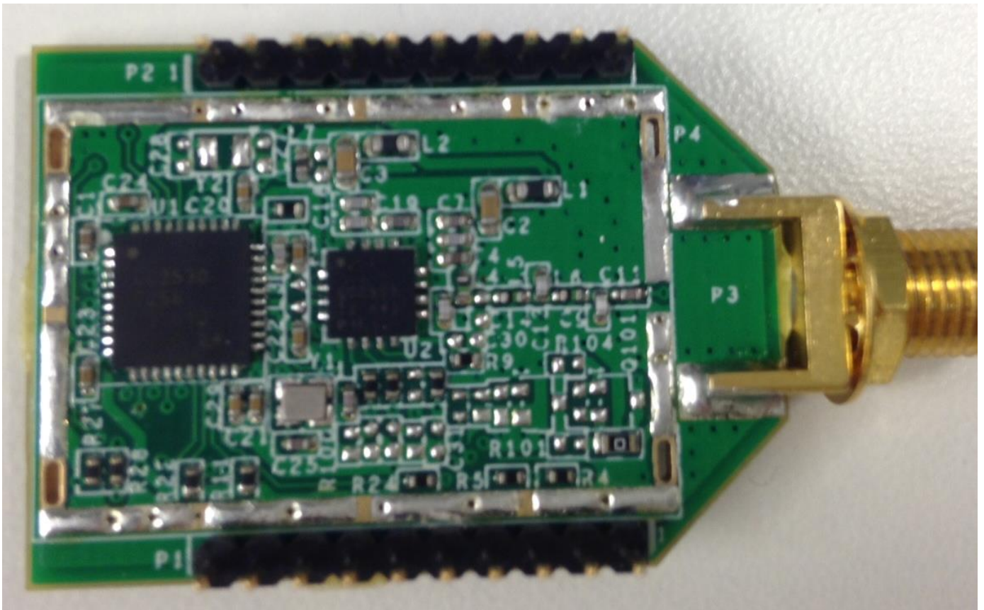
(EUT Bottom)
