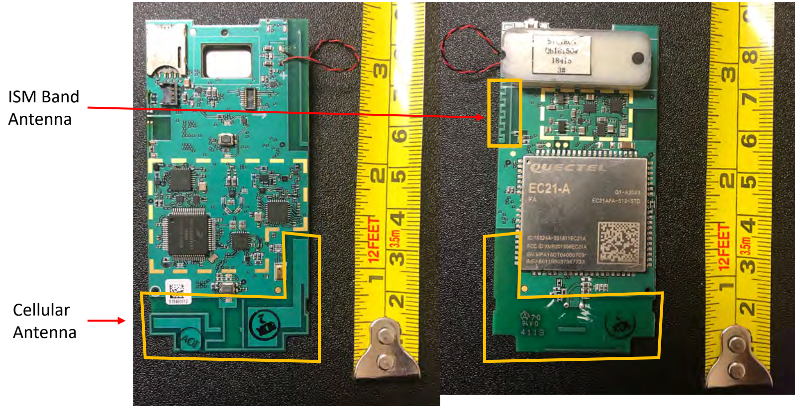
PCA Top
