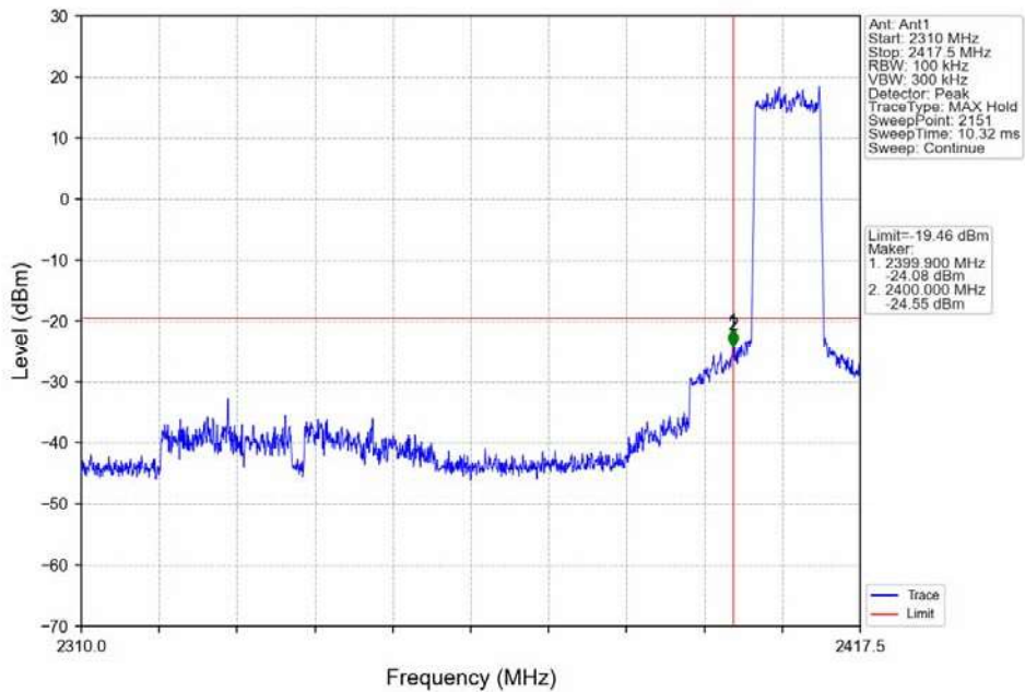
QPSK 10MHz_LCH_2407.5MHz_Ant1_NTNV
