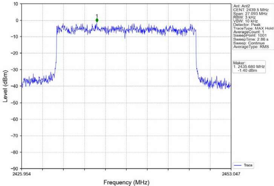
16QAM 20MHz_MCH_2439.5MHz_Ant2_NTNV
