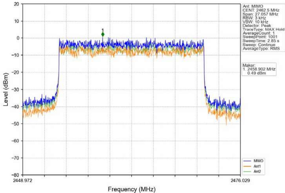
16QAM 20MHz_HCH_2462.5MHz_MIMO_NTNV
