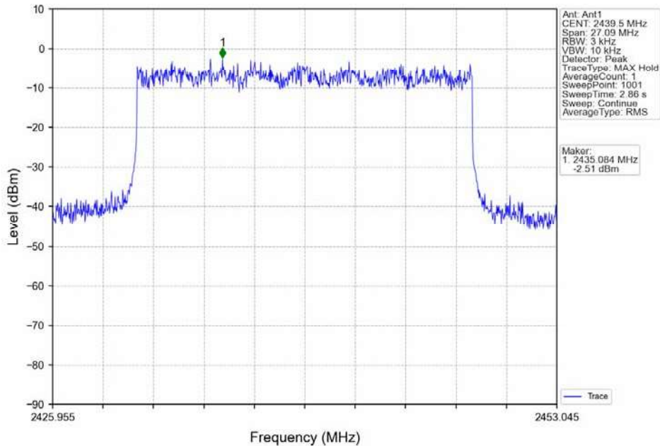
QPSK 20MHz_MCH_2439.5MHz_Ant1_NTNV
