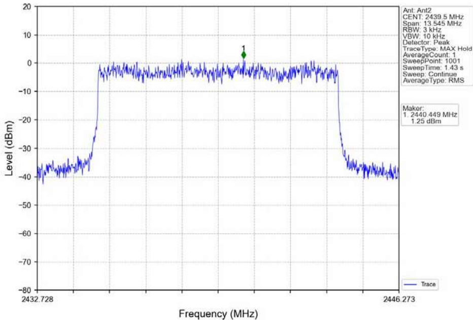
16QAM 10MHz_MCH_2439.5MHz_Ant2_NTNV
