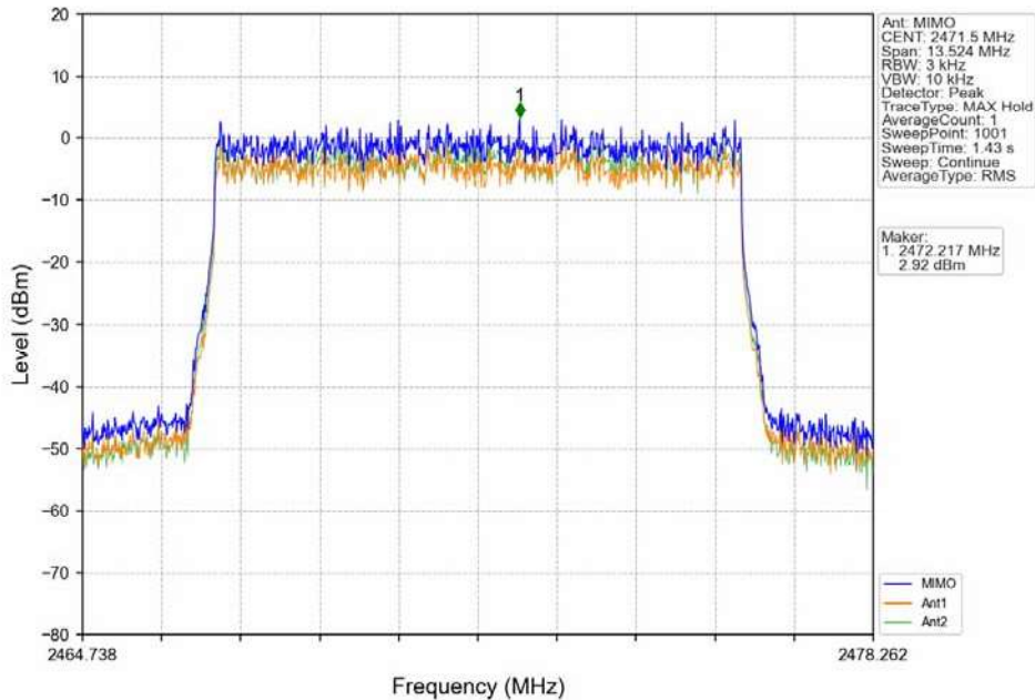
16QAM 10MHz_HCH_2471.5MHz_MIMO_NTNV
