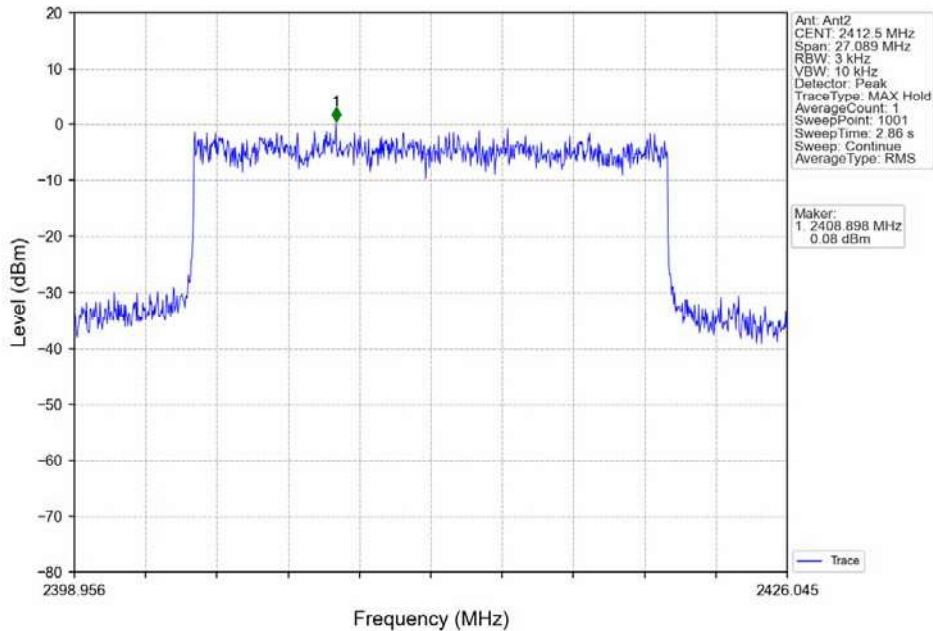
QPSK 20MHz_LCH_2412.5MHz_Ant2_NTNV
