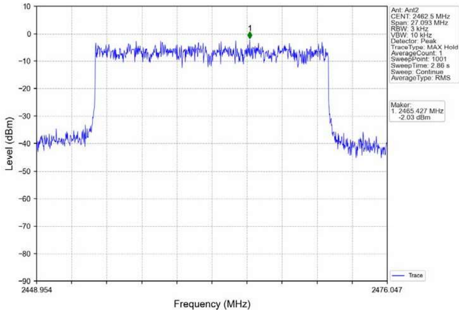
QPSK 20MHz_HCH_2462.5MHz_Ant2_NTNV
