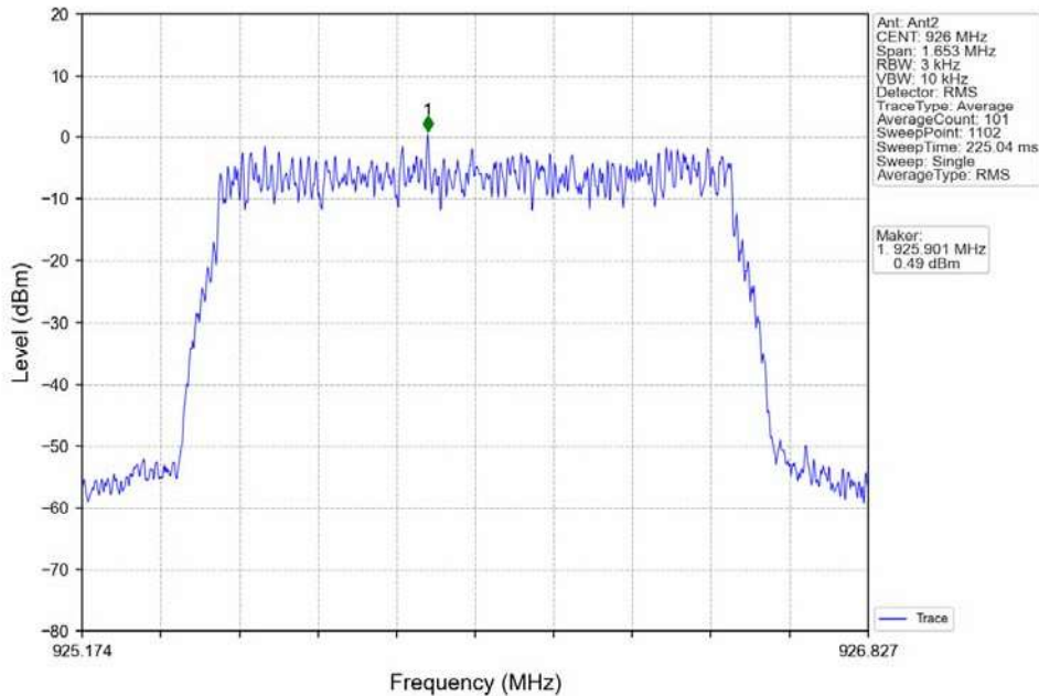
QPSK 1.4MHz_HCH_926MHz_Ant2_NTNV
