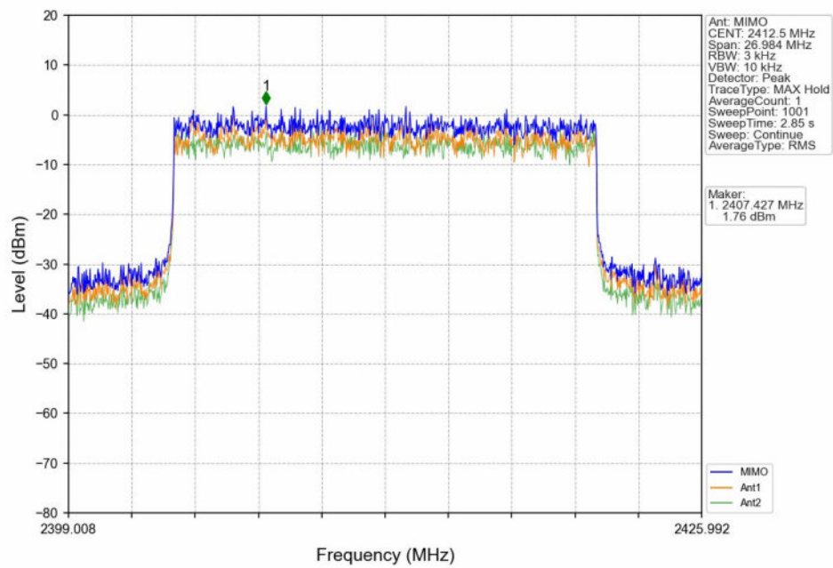
16QAM_LCH_2412.5MHz_MIMO_NTNV
