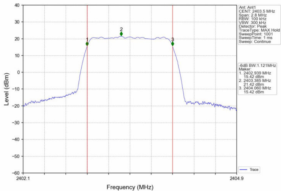
16QAM_LCH_2403.5MHz_MIMO_NTNV
