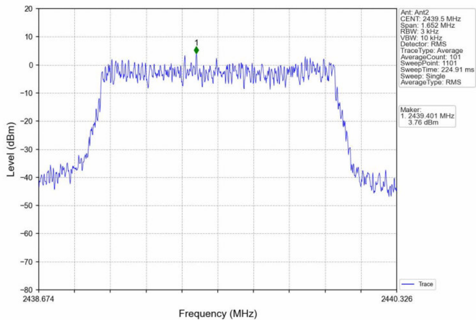
16QAM_MCH_2439.5MHz_Ant2_NTNV
