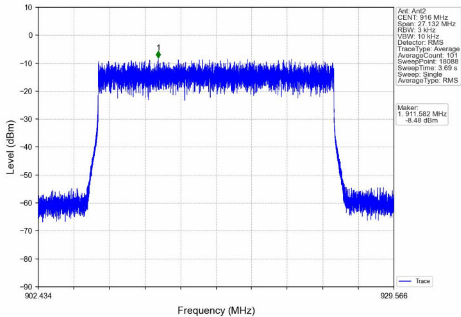
16QAM_HCH_916MHz_MIMO_NTNV
