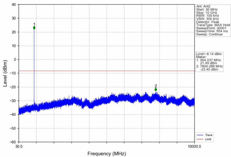
QPSK_LCH_904MHz_Ant2_NTNV
