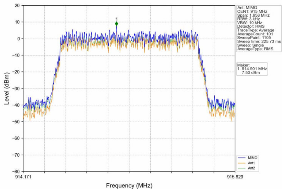
QPSK_MCH_915MHz_MIMO_NTNV
