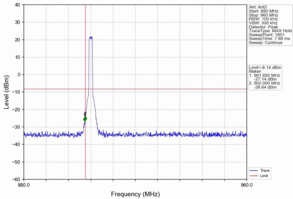
QPSK_LCH_904MHz_Ant2_NTNV
