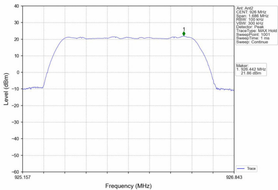
16QAM_HCH_926MHz_Ant2_NTNV
