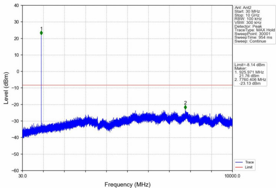
16QAM_HCH_926MHz_Ant2_NTNV
