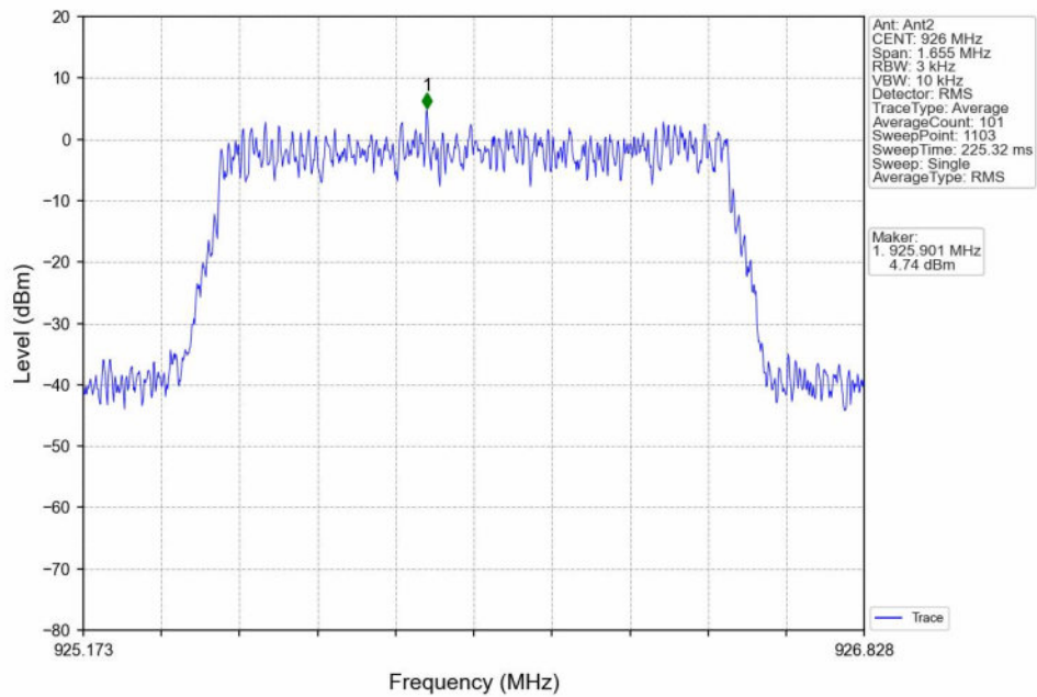
16QAM_HCH_926MHz_MIMO_NTNV
