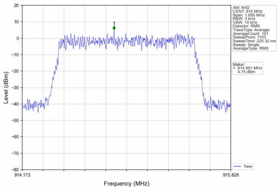
16QAM_MCH_915MHz_Ant2_NTNV
