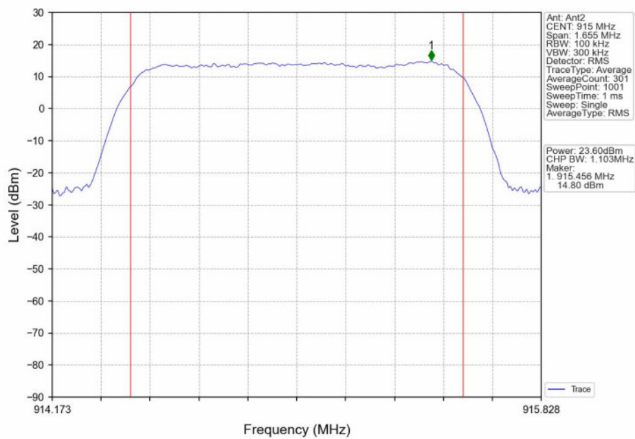
16QAM_MCH_915MHz_Ant2_NTNV
