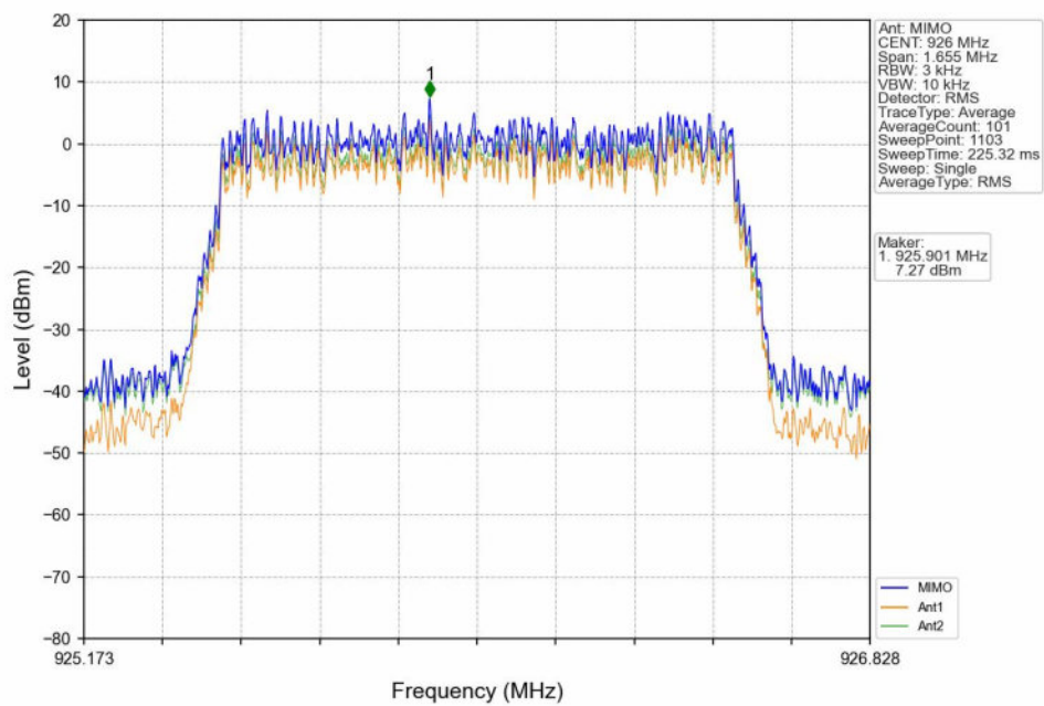
16QAM_HCH_926MHz_MIMO_NTNV
