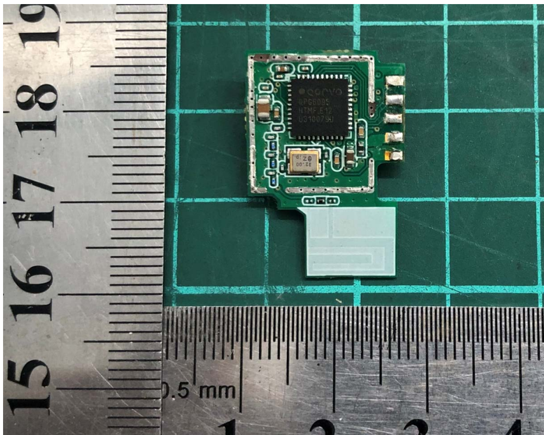
a: EUT
