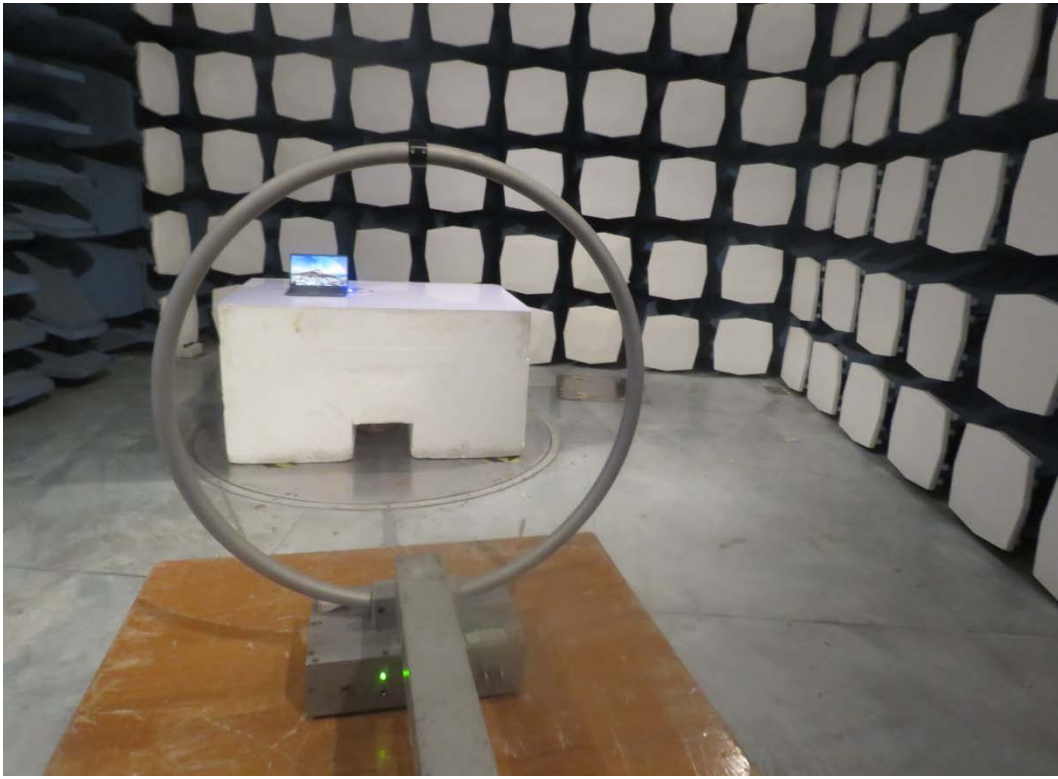
9kHz-30MHz
