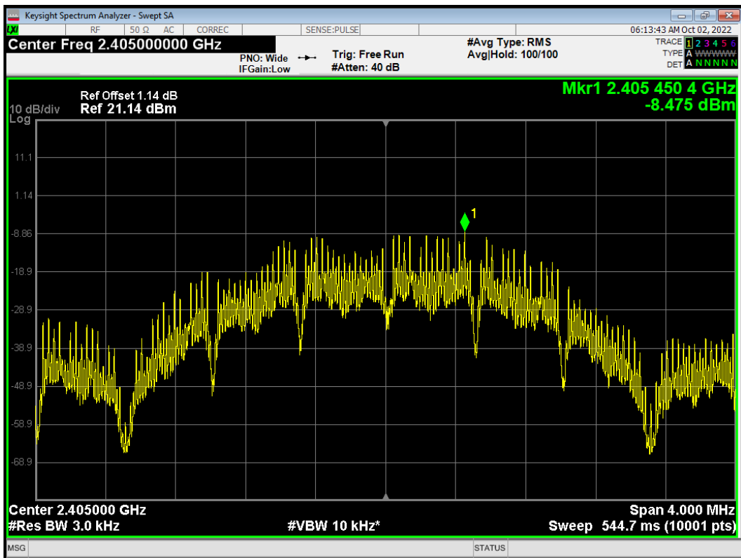
PSD ZigBee 2405MHz
