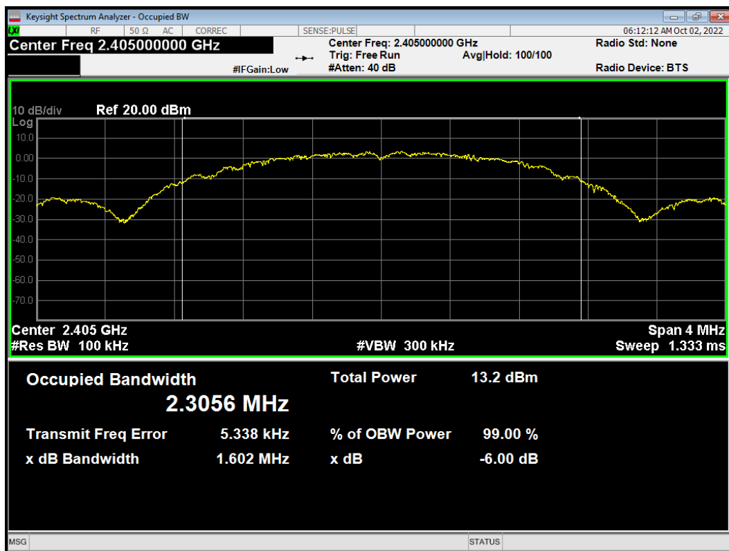
-6dB Bandwidth ZigBee 2405MHz
