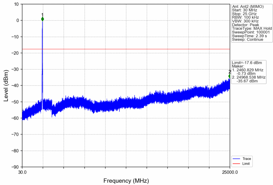
802.11ax(HEW40)_HCH_2452MHz_RU484_Left_Ant2 (MIMO)_NTNV
