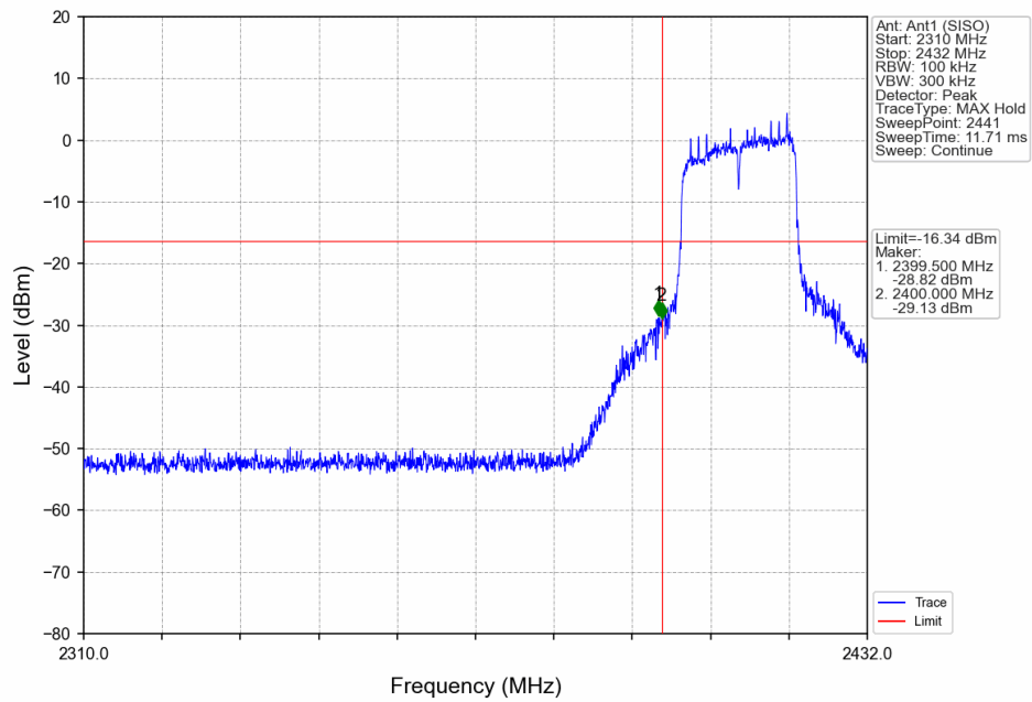
802.11ax(HEW20)_LCH_2412MHz_RU242_Left_Ant1 (SISO)_NTNV
