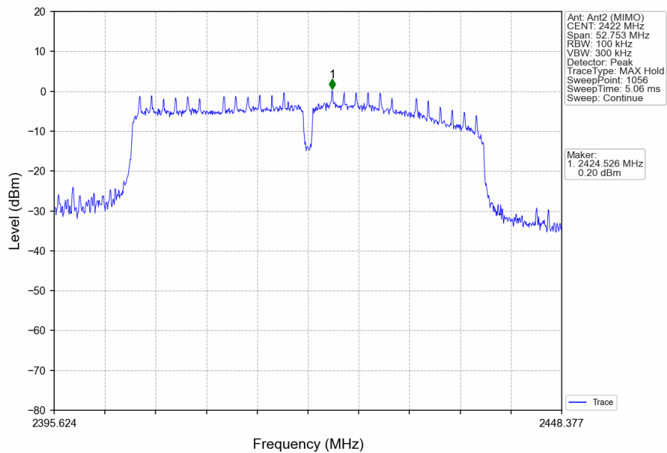
802.11ax(HEW40)_LCH_2422MHz_RU484_Left_Ant2 (MIMO)_NTNV
