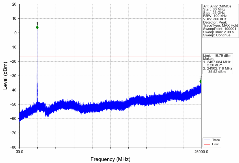
802.11ax(HEW20)_HCH_2462MHz_RU242_Left_Ant2 (MIMO)_NTNV
