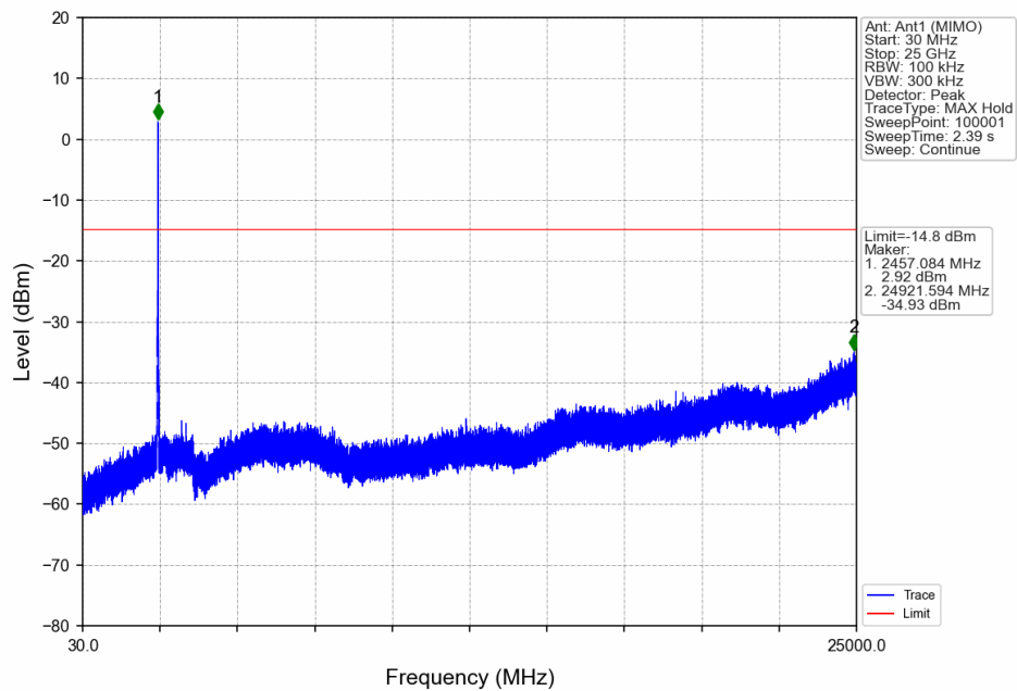
802.11ax(HEW20)_HCH_2462MHz_RU242_Left_Ant1 (MIMO)_NTNV
