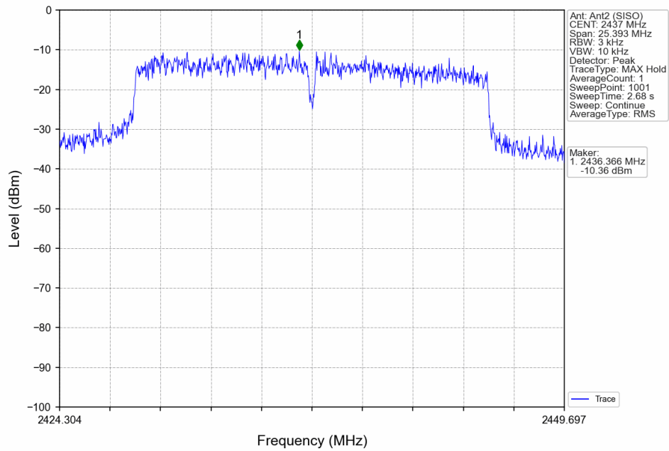
802.11ax(HEW20)_MCH_2437MHz_RU242_Left_Ant2 (SISO)_NTNV
