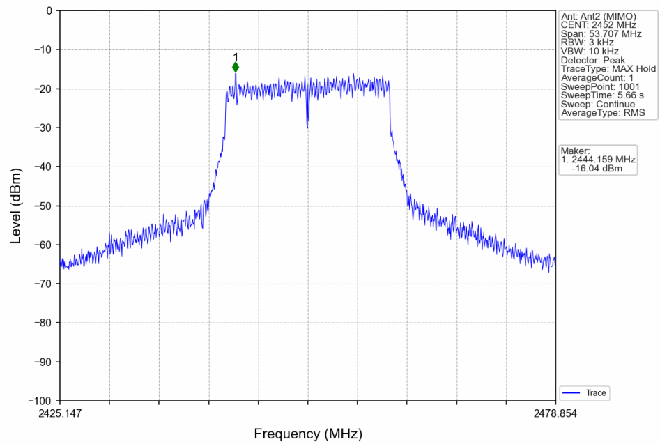
802.11n(HT40)_HCH_2452MHz_MIMO_NTNV
