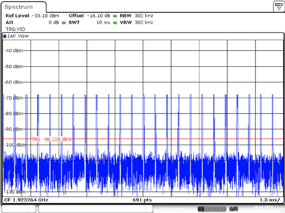
35 µs Pulses
