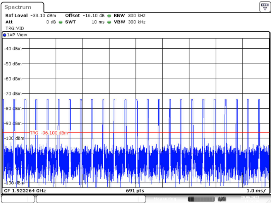
50 µs Pulses
