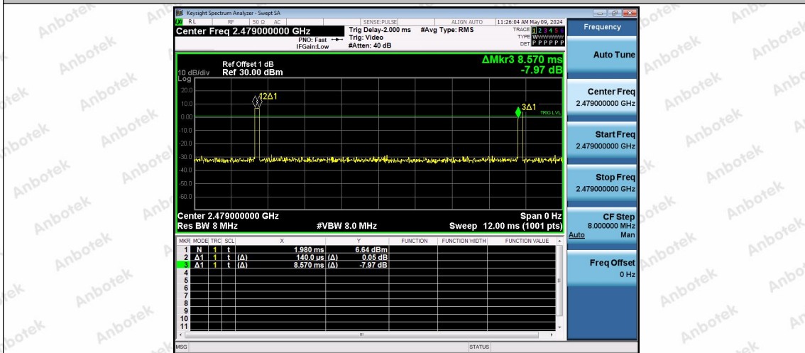
NTNV-2.4G-Ant1-2479
