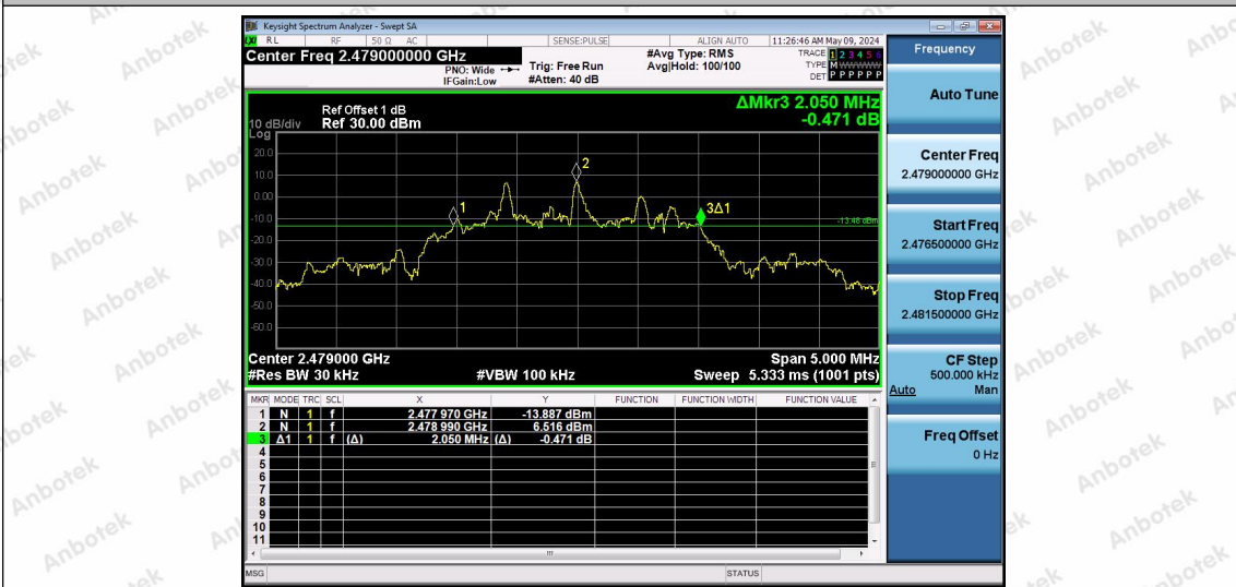
2.4G-Ant1-2479
