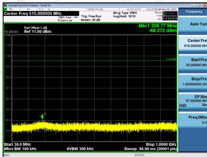
2.4G-Ant1-2403-30~1000-PASS
