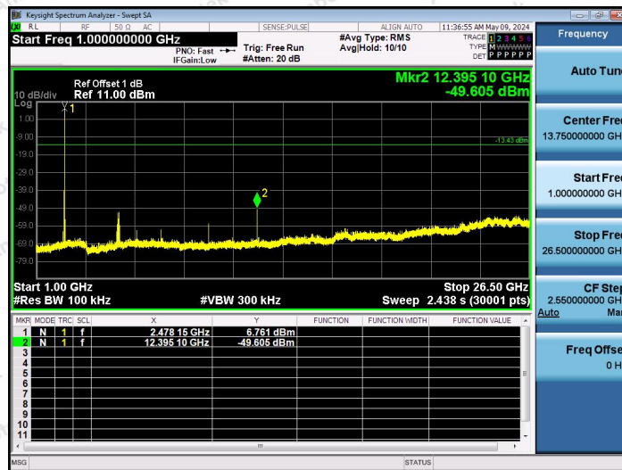
2.4G-Ant1-2479-1000~26500-PASS
