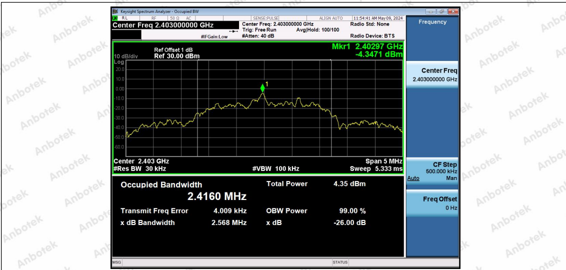
2.4G-Ant1-2403
