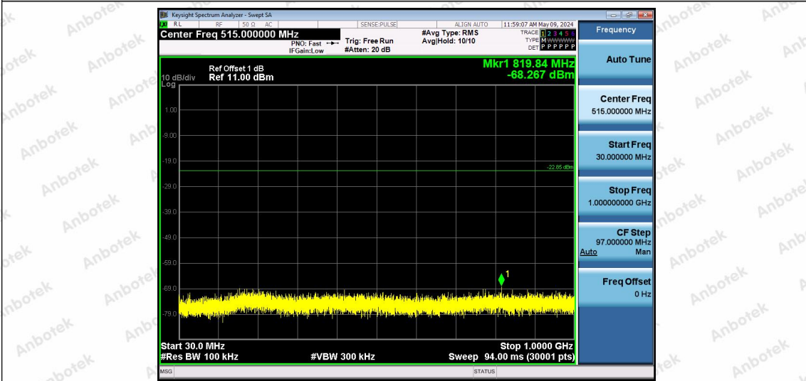
2.4G-Ant1-2403-30~1000-PASS
