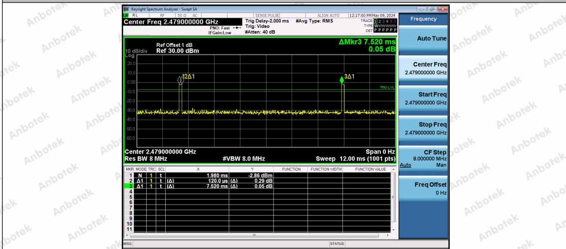
NTNV-2.4G-Ant1-2479
