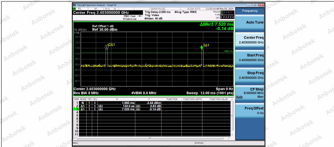
NTNV-2.4G-Ant1-2403
