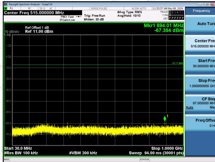
2.4G-Ant1-2479-30~1000-PASS
