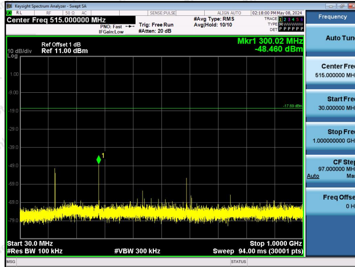
2.4G-Ant1-2474-30~1000-PASS
