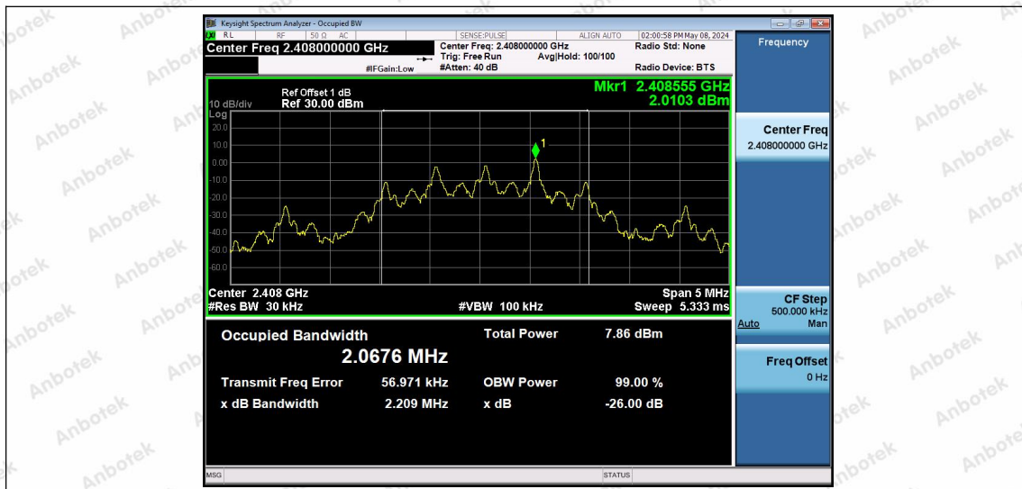
2.4G-Ant1-2408
