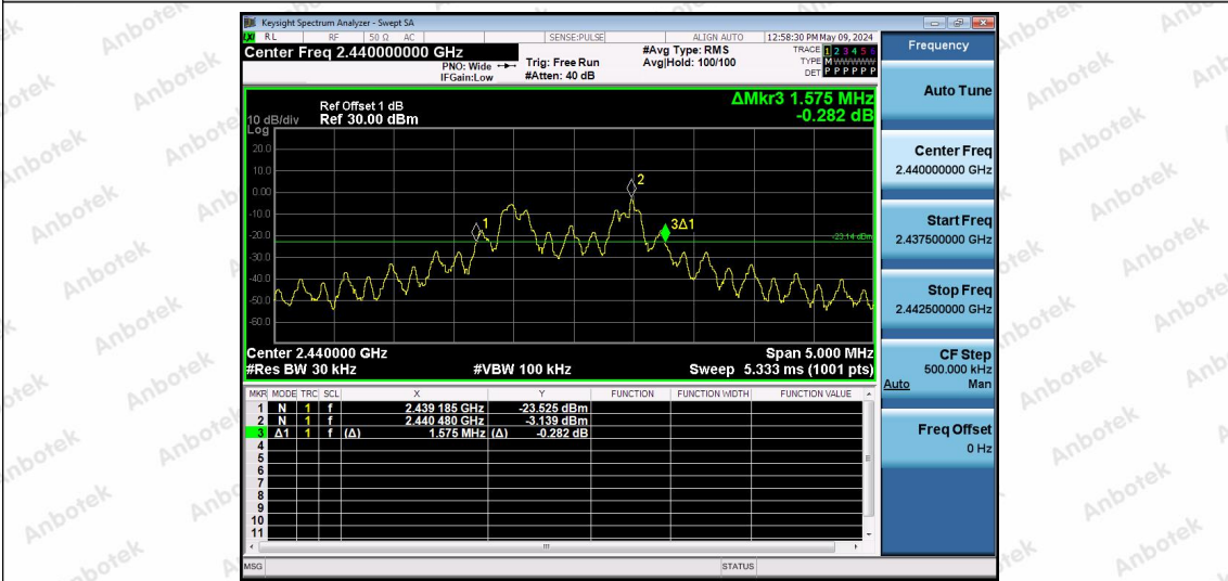
2.4G-Ant1-2440
