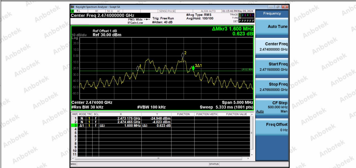
2.4G-Ant1-2474
