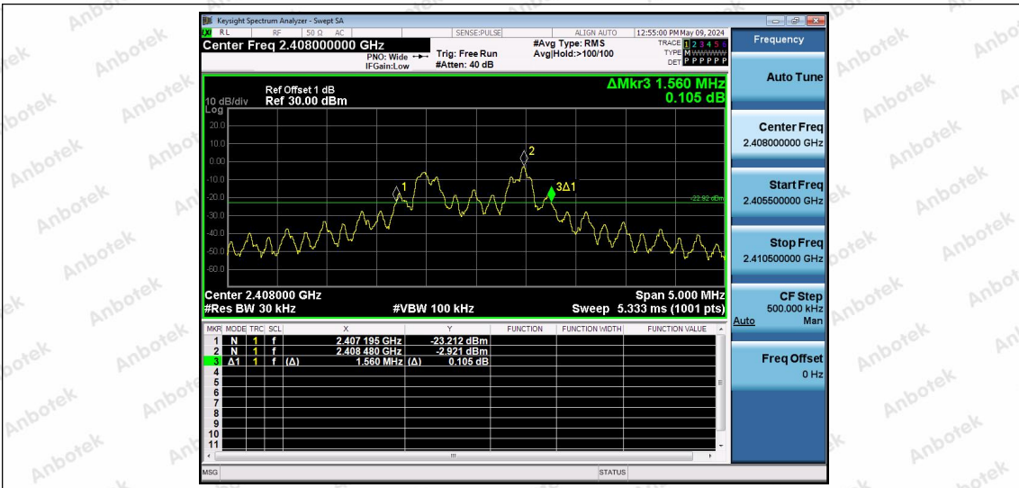
2.4G-Ant1-2408
